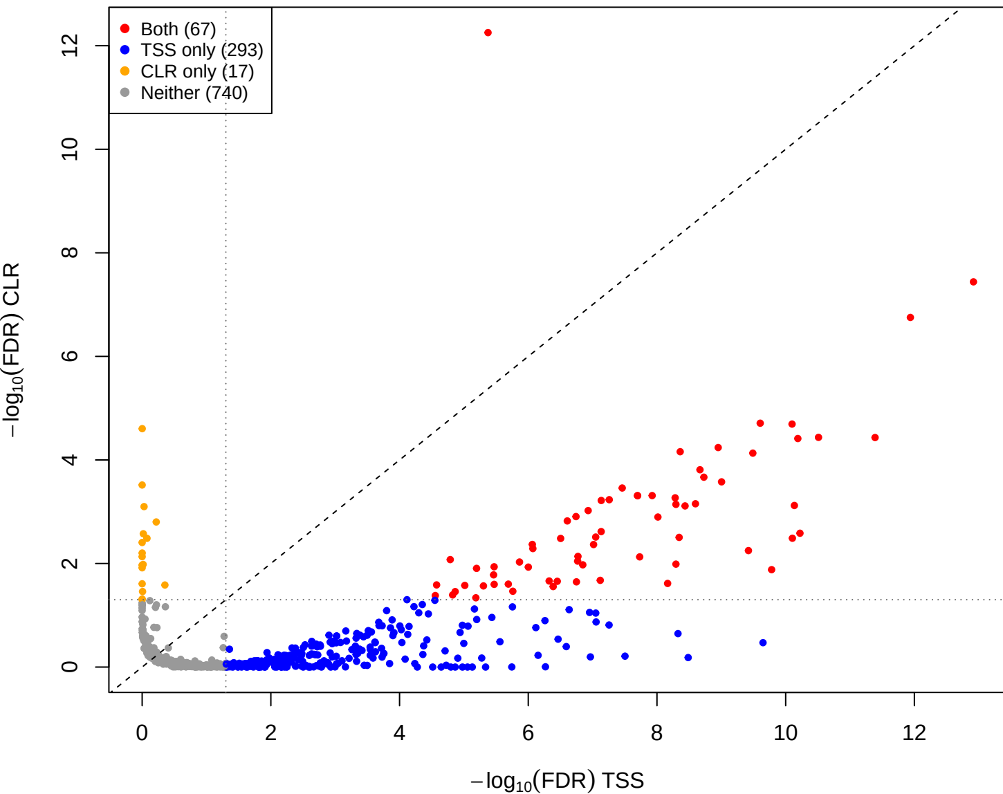
mage vs mid - CLR vs TSS(const=1) (gamma = 1e-05)
