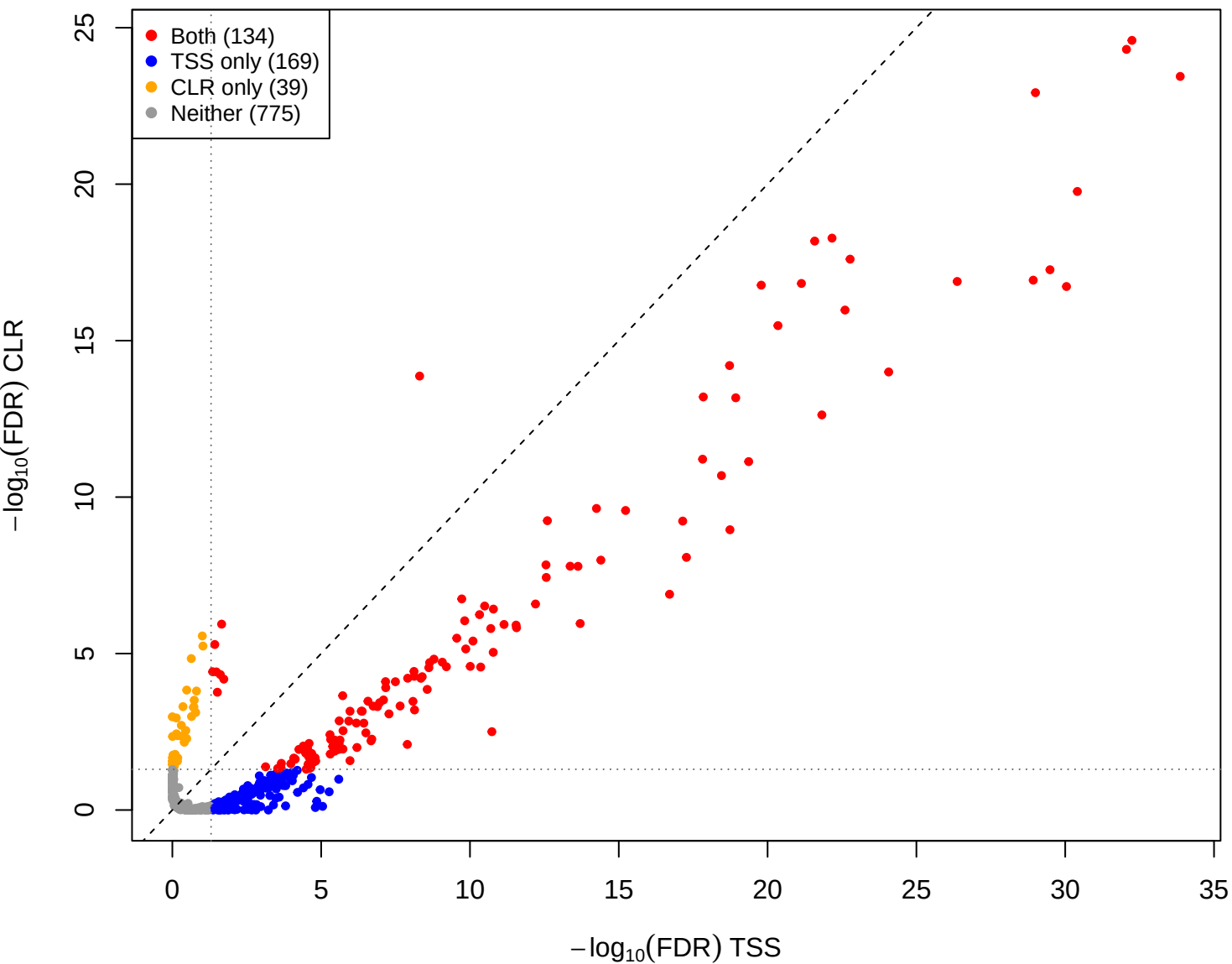
eld vs mid – CLR vs TSS(const=1) (gamma = 1e-05)
