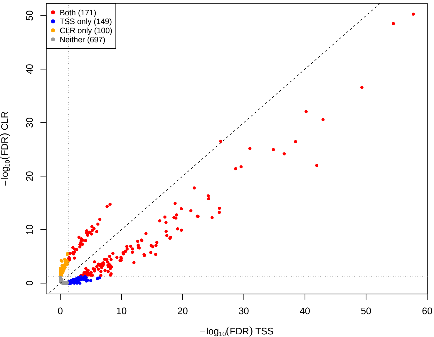
cent vs kin - CLR vs TSS(const=1) (gamma = 1e-05)
