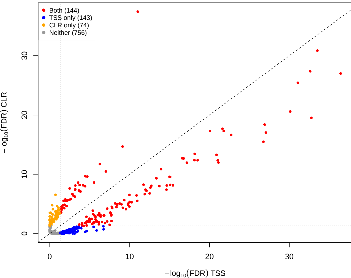
eld vs kin – CLR vs TSS(const=1) (gamma = 1e-05)
