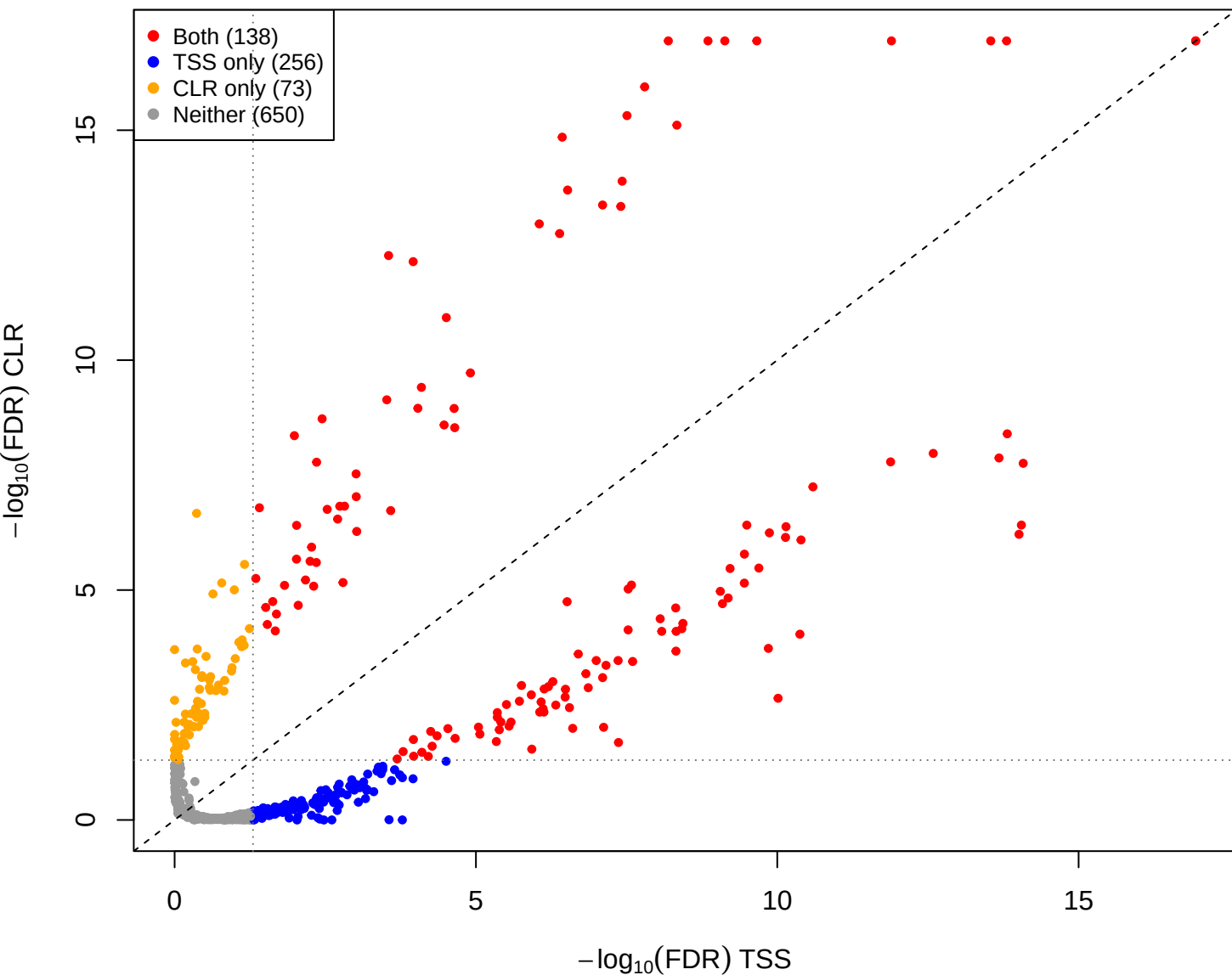
mage vs you - CLR vs TSS(const=1) (gamma = 1e-05)
