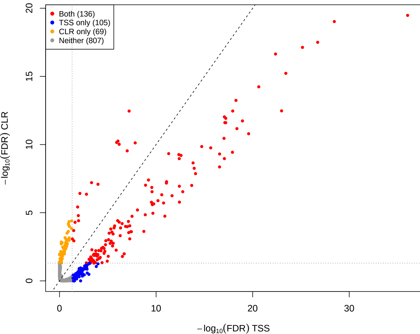
cent vs mage – CLR vs TSS(const=1) (gamma = 1e-05)
