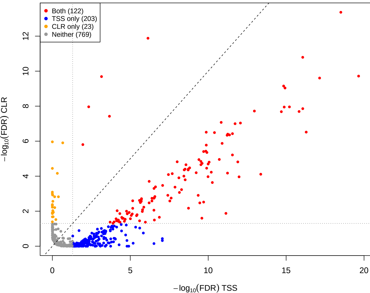
kin vs mid – CLR vs TSS(const=1) (gamma = 1e-05)
