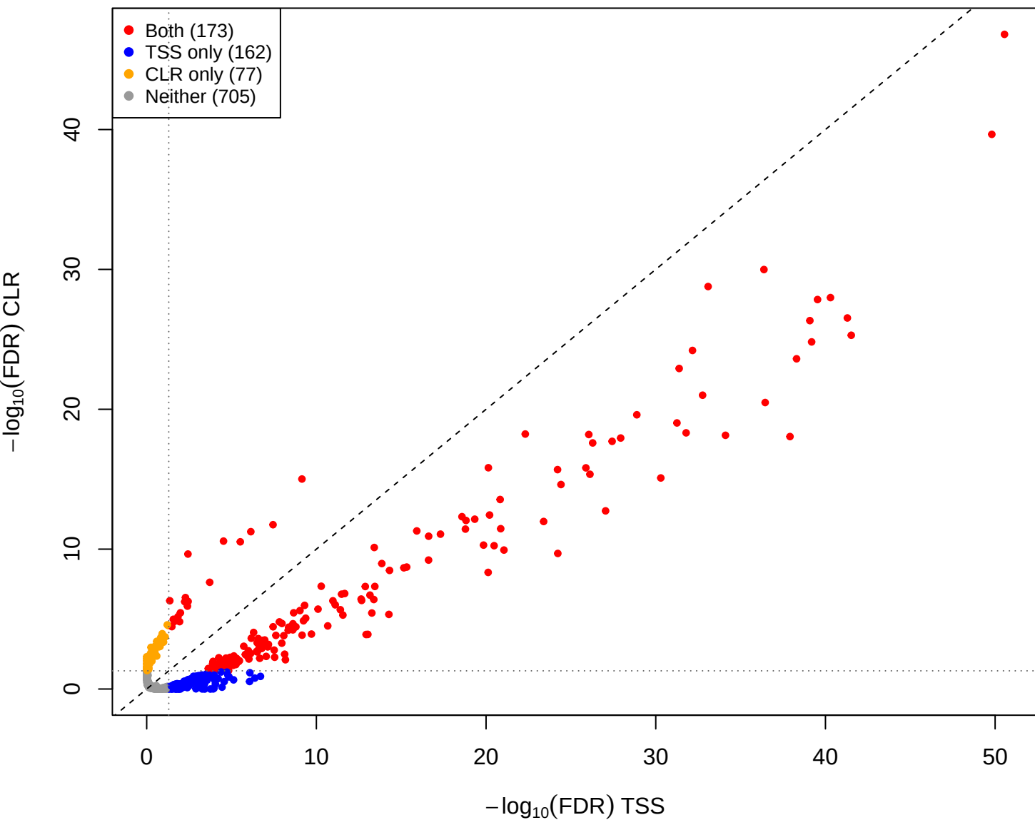
cent vs mid – CLR vs TSS(const=1) (gamma = 1e-05)
