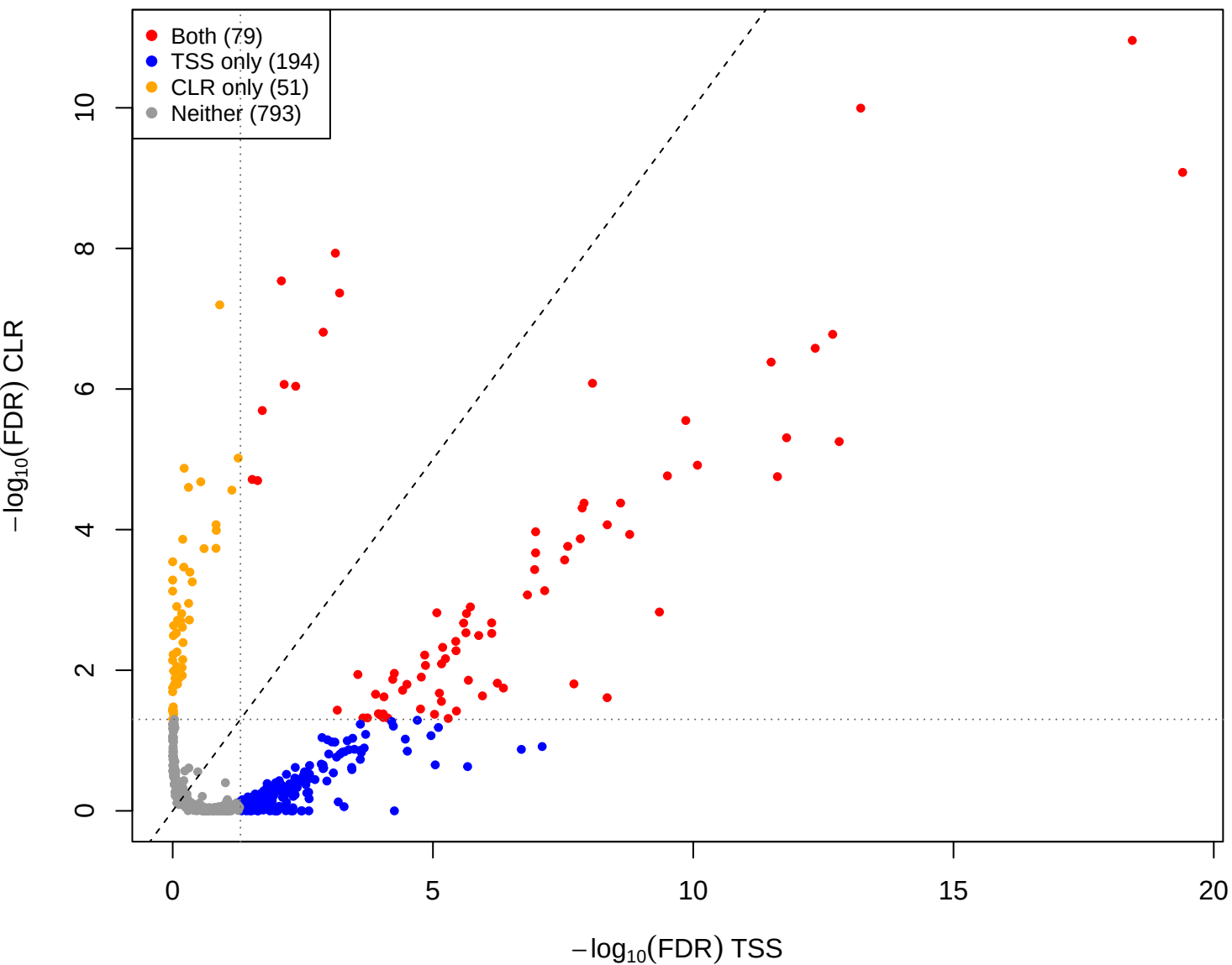
cent vs eld - CLR vs TSS(const=1) (gamma = 1e-05)
