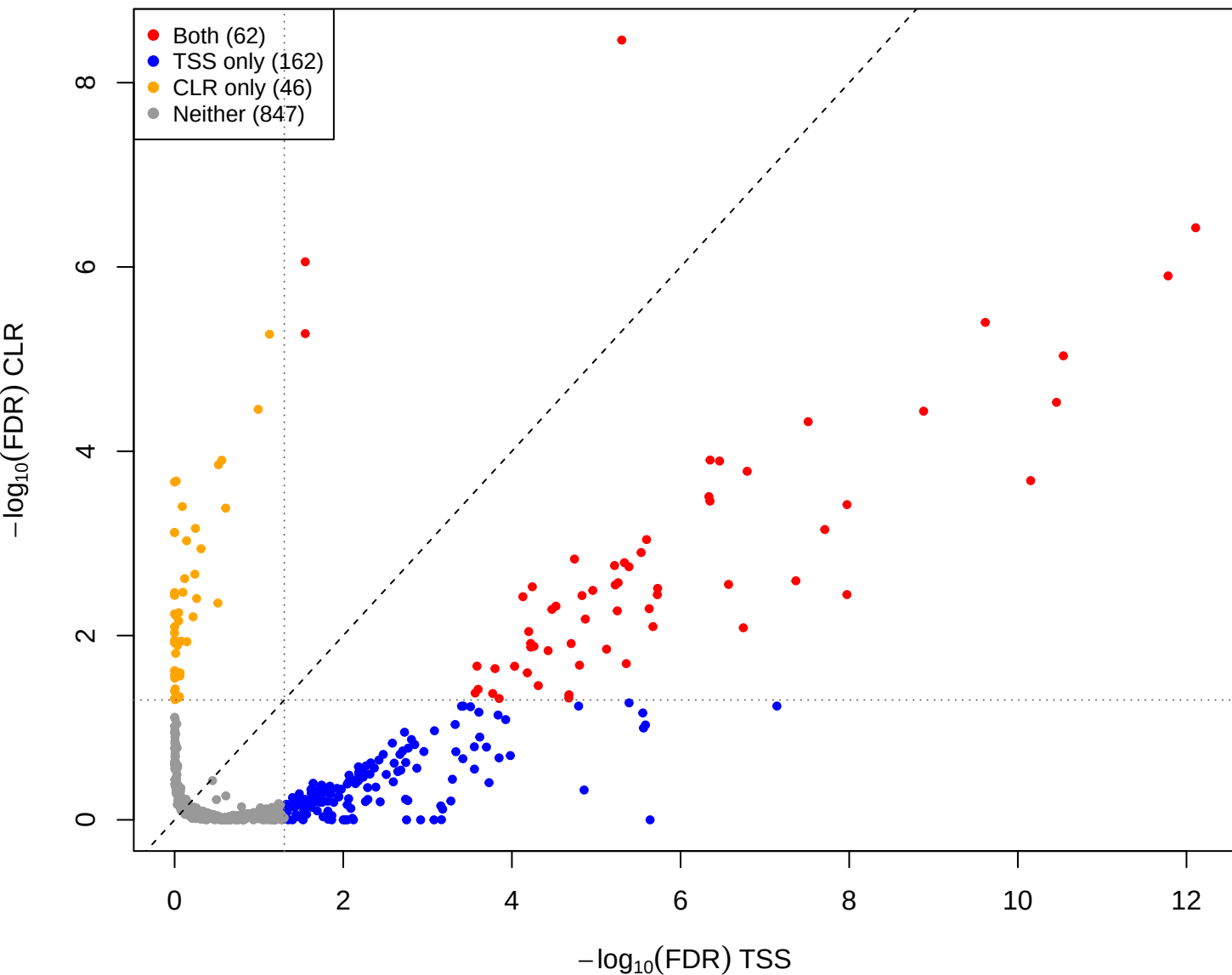
kin vs mage – CLR vs TSS(const=1) (gamma = 1e-05)
