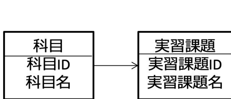
ER図
