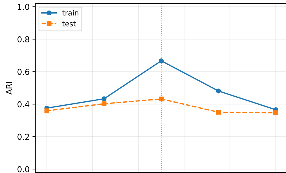
mnist
