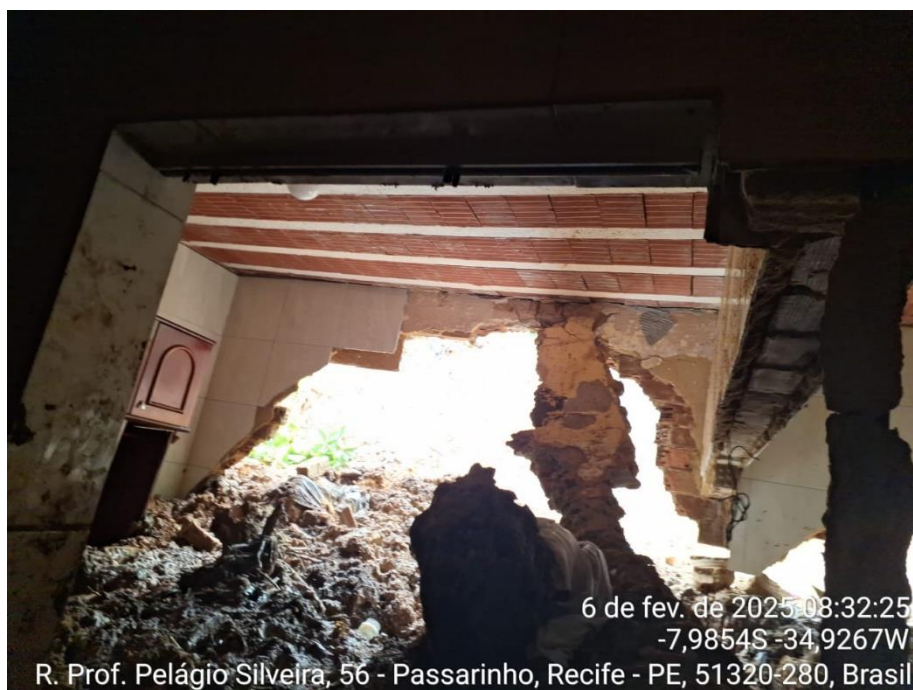
Figura 4- cômodo adjacente ao da figura anterior em condição semelhante.
