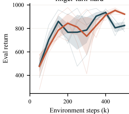
finger-turn-hard
