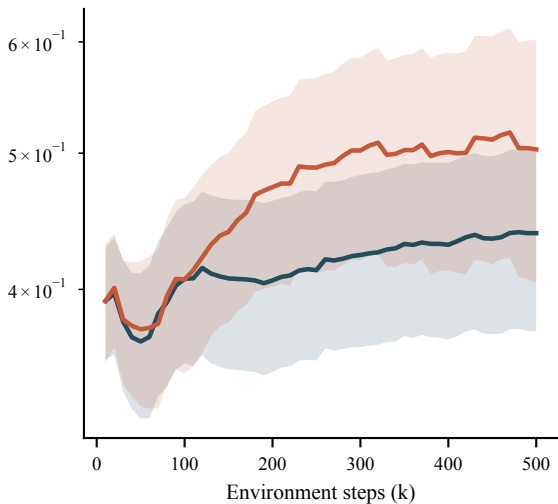
Gradient norm
