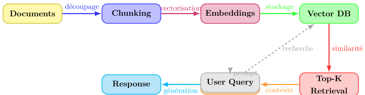
FIGURE 3.4 – Pipeline RAG : indexation, vectorisation, récupération et génération
