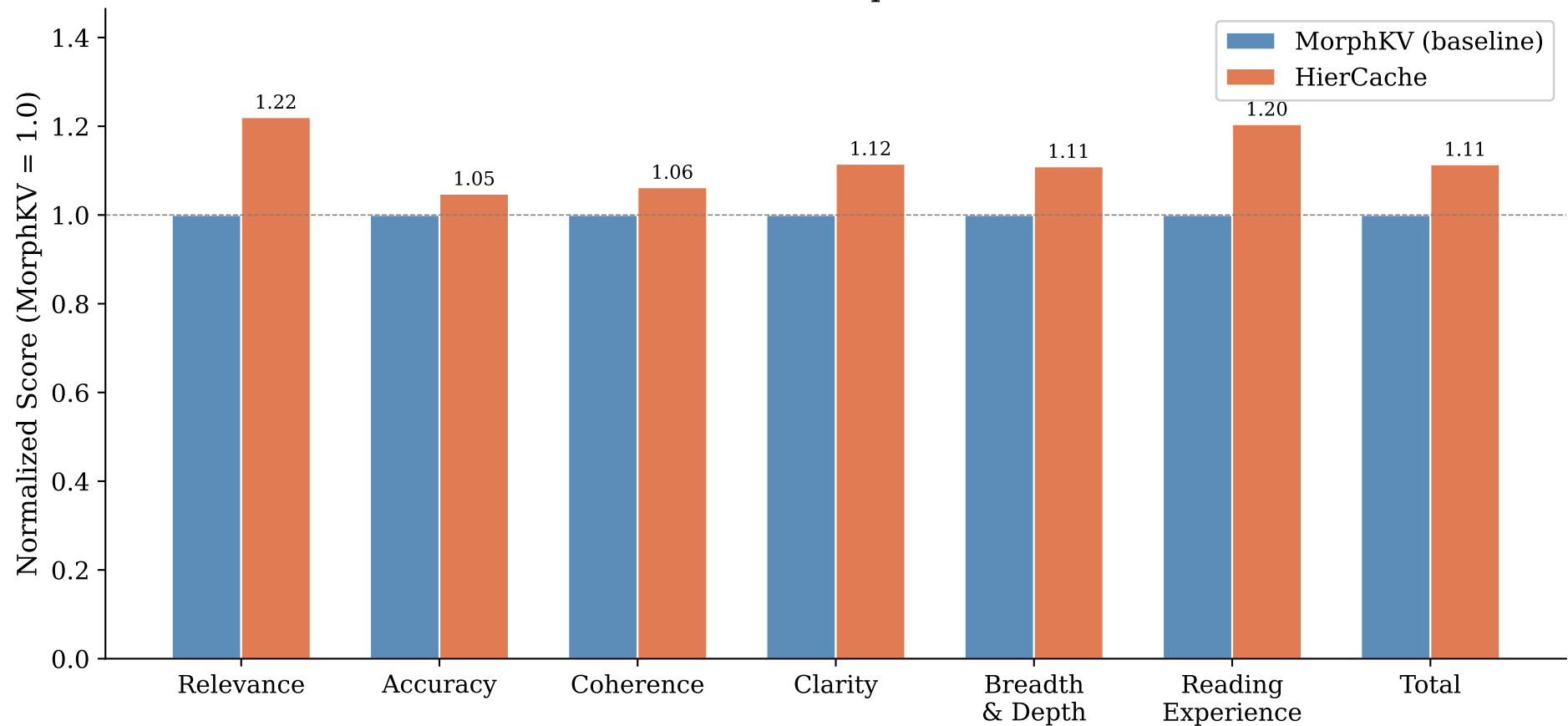
HierCache vs MorphKV — Phi-4
