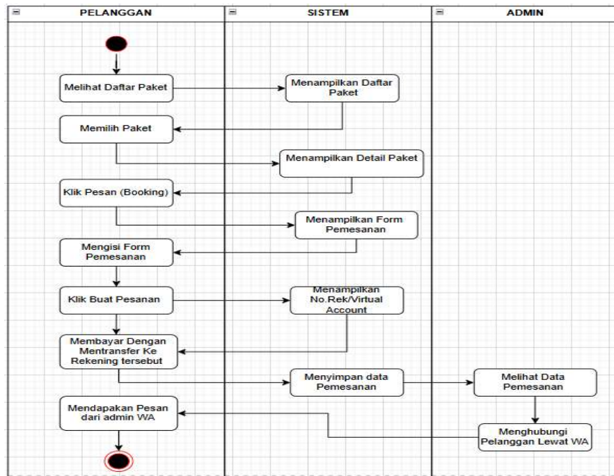
Gambar 3.2.2 Activity Diagram Pemesanan
