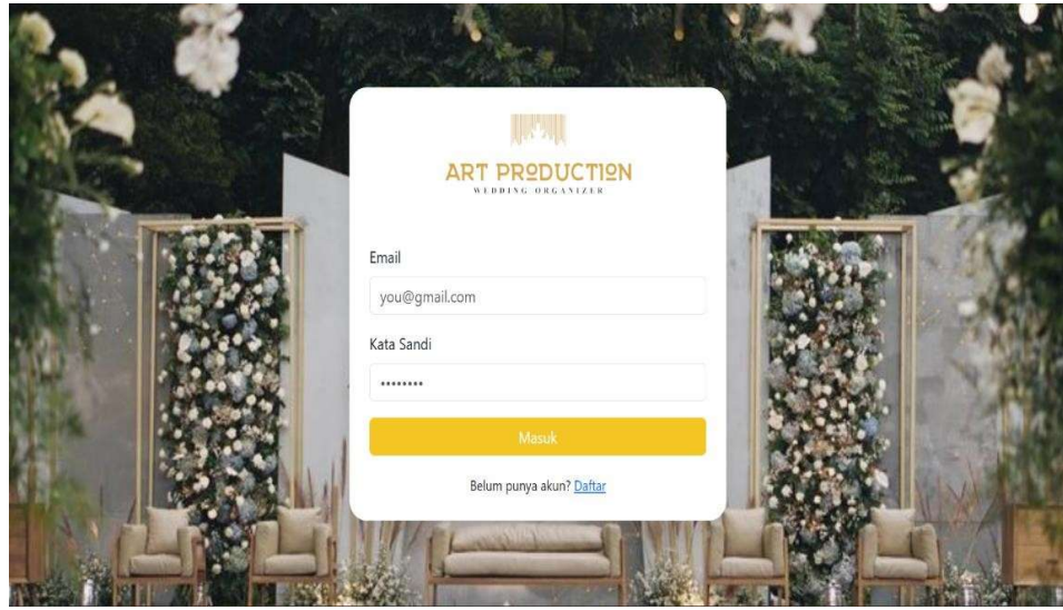
Gambar 4.1.1 Login
