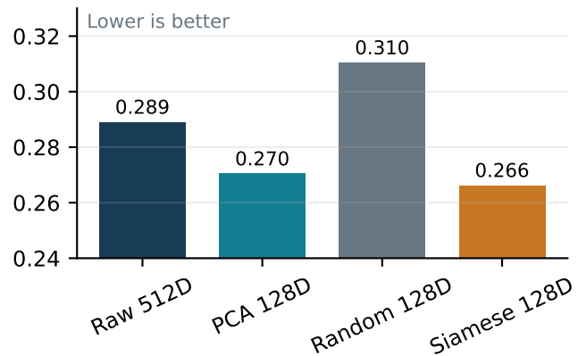
EER
