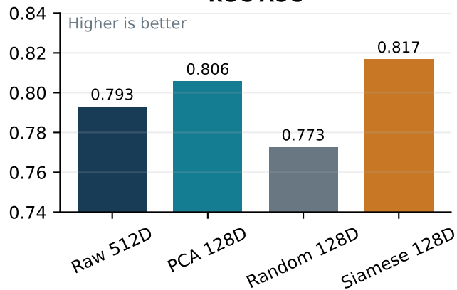
ROC AUC
