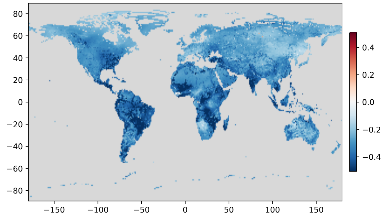
R^2
