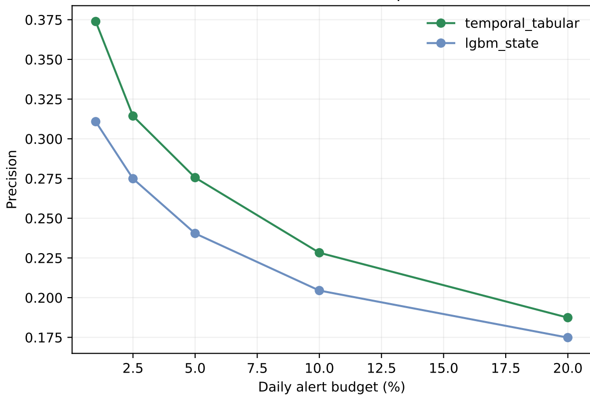
2025: session-level alert precision
