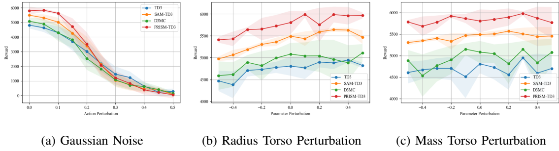
Fig. 2: Ant-v4
