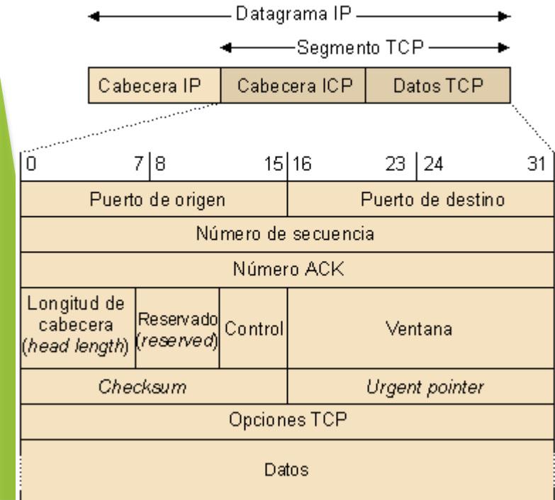
Segmento TCP
