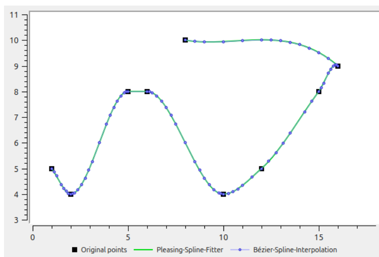
Abbildung 89. SplineLocal: generiert mittels polygon() und mittels painterPath()
