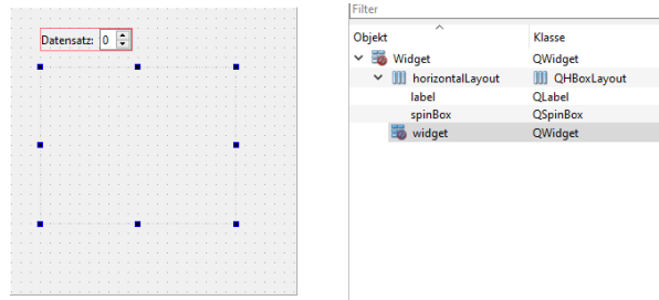
Abbildung 91. Widget mit Platzhalter-Widget für das Diagramm
