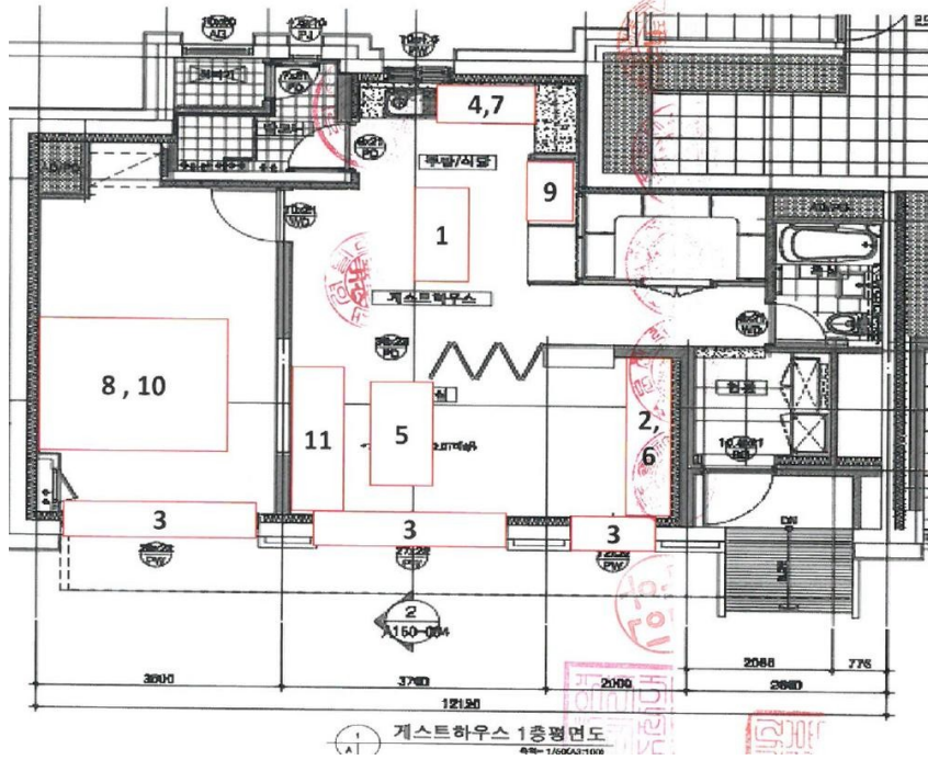
게스트하우스 1층 평면도 — 번호는 위 수량표의 품목 번호 (조사보고서)
