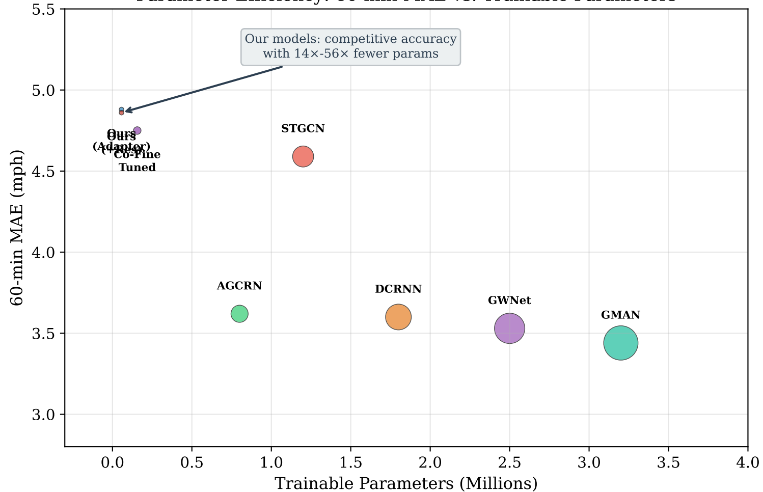
Parameter Efficiency: 60-min MAE vs. Trainable Parameters
