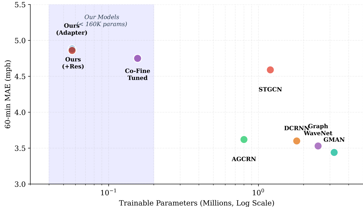
Parameter Efficiency: 60-min MAE vs. Parameters
