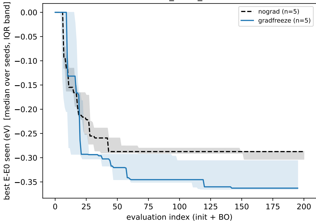
ML0_3HF8_A
