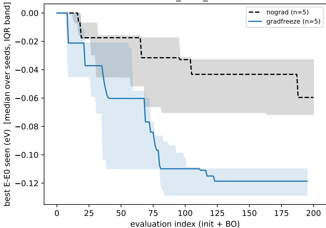
RO7_3G8I_A
