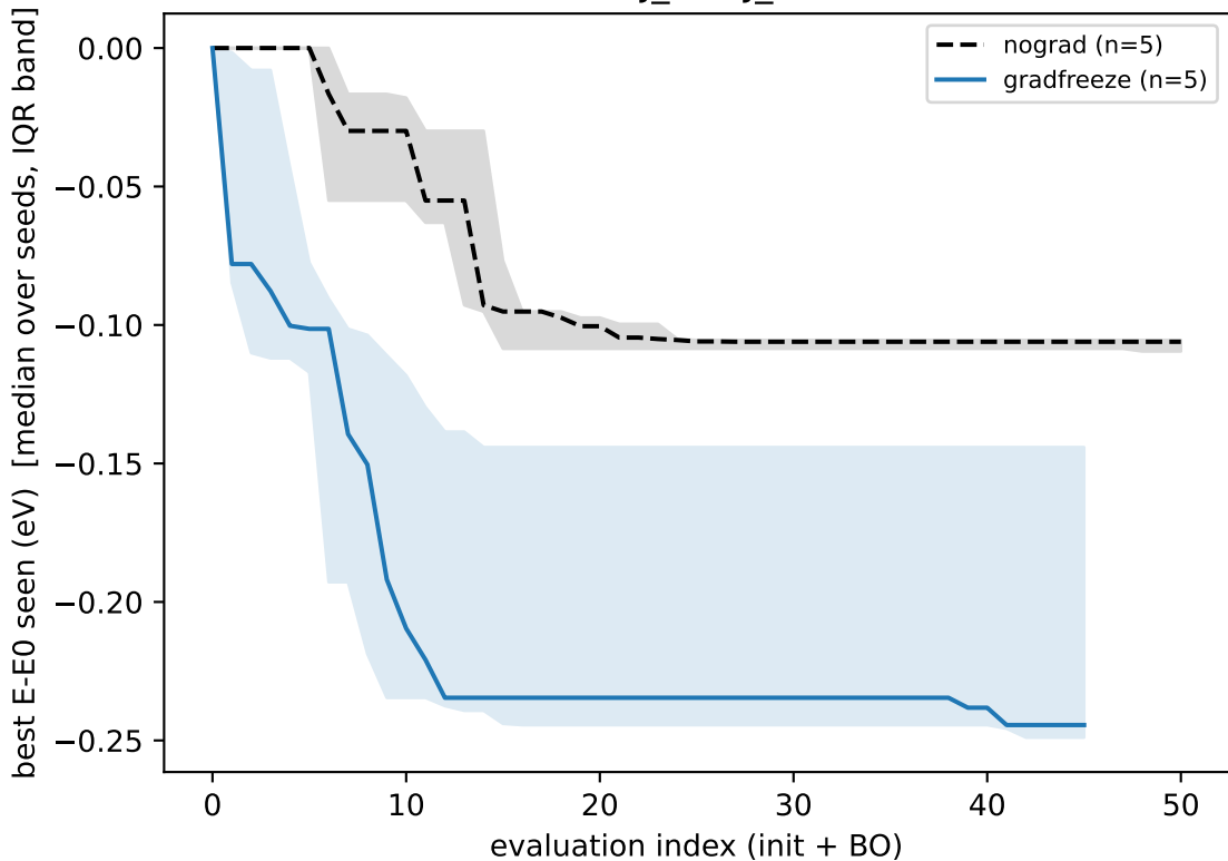
4EJ_4YMJ_A
