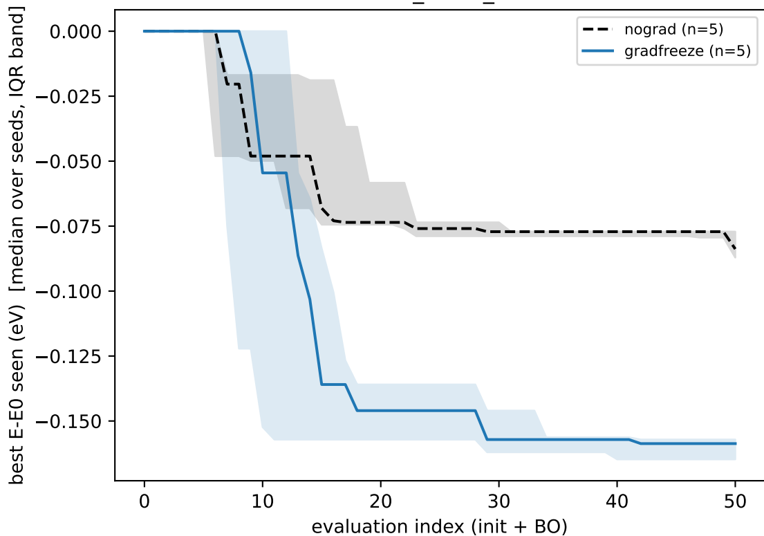
BP5_2PXH_A
