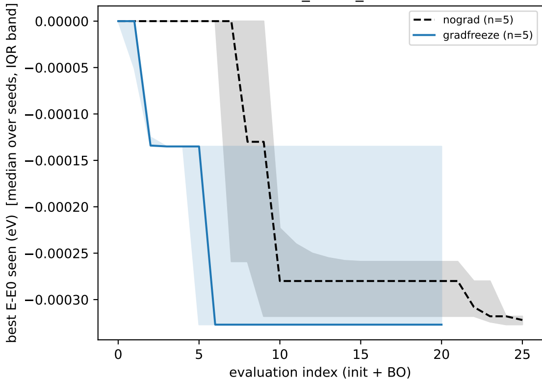
ORO_3ZWT_A
