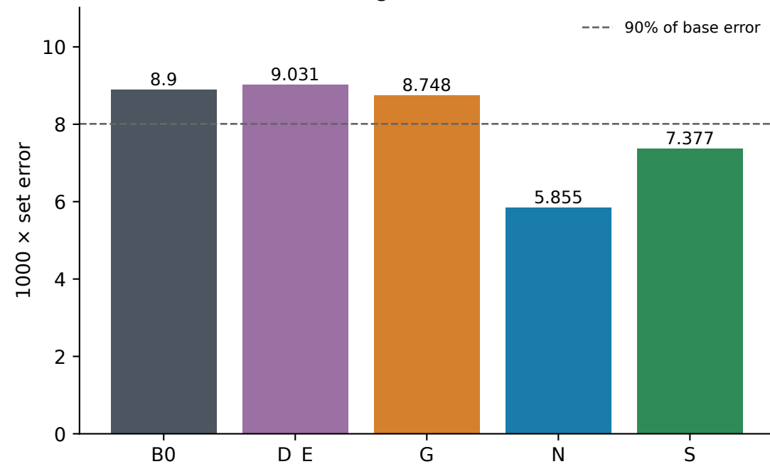
(d) Physical qualification is separate
