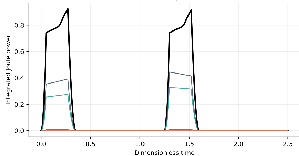
(d) Joule response
