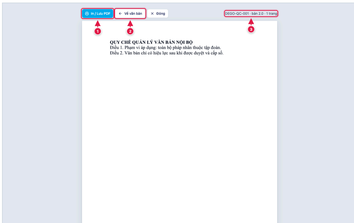
Hình 37. Trang in
