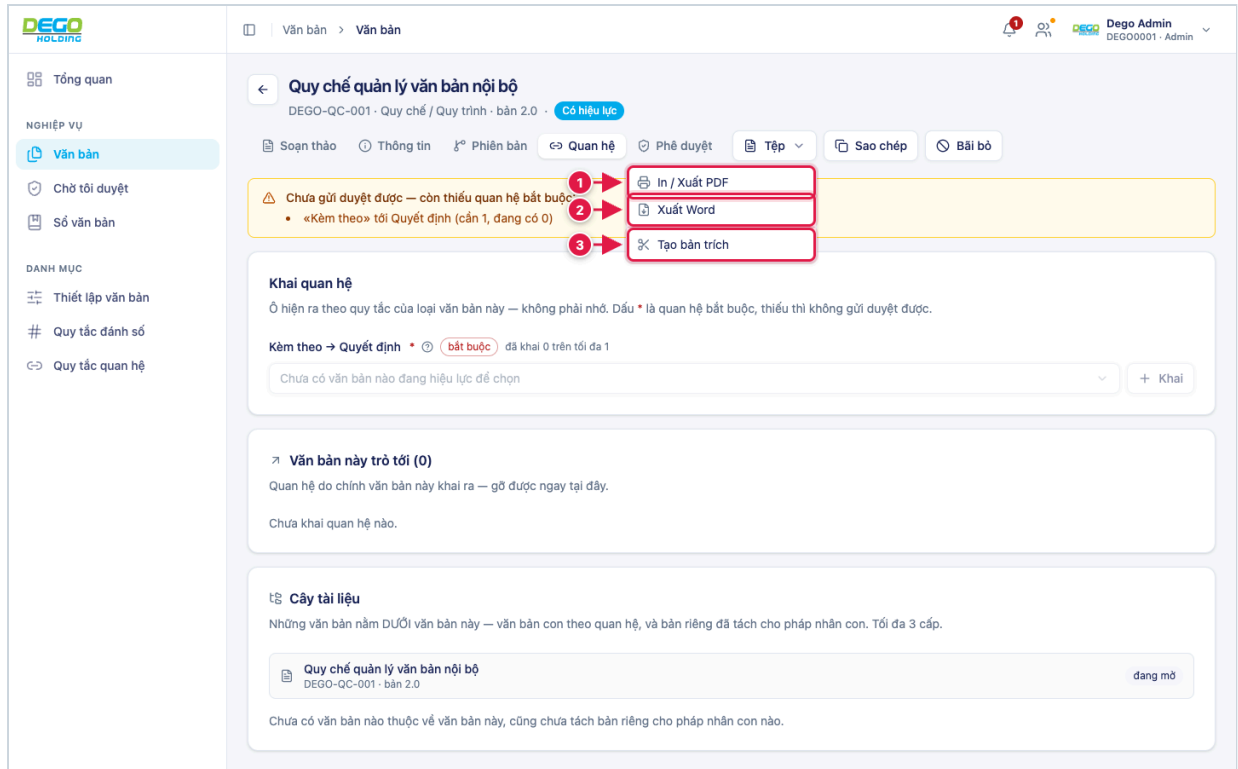
Hình 36. Menu Tập
