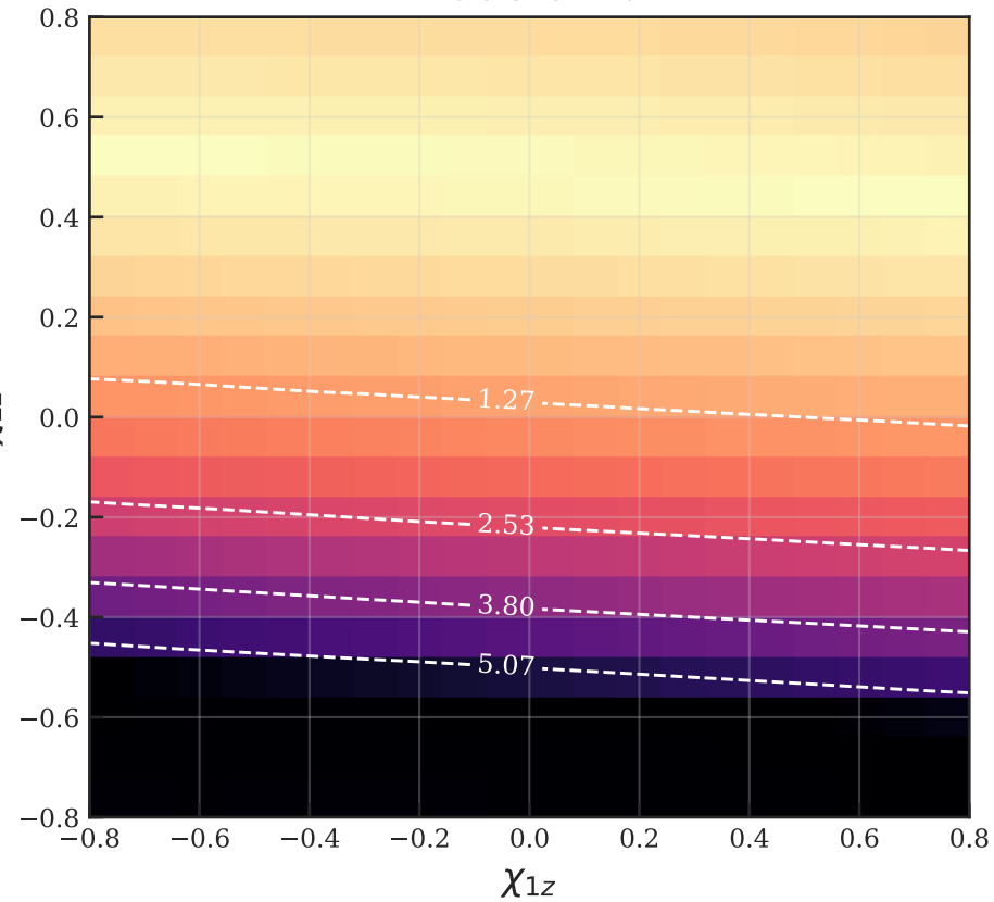
Padé 0PN
