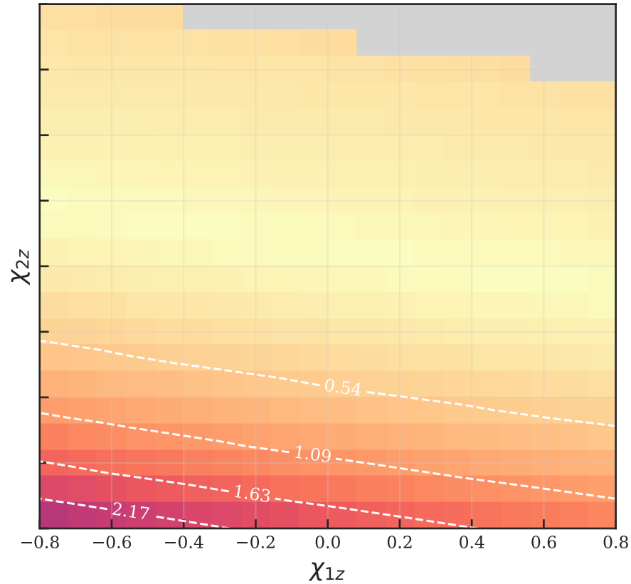
Padé 1PN
