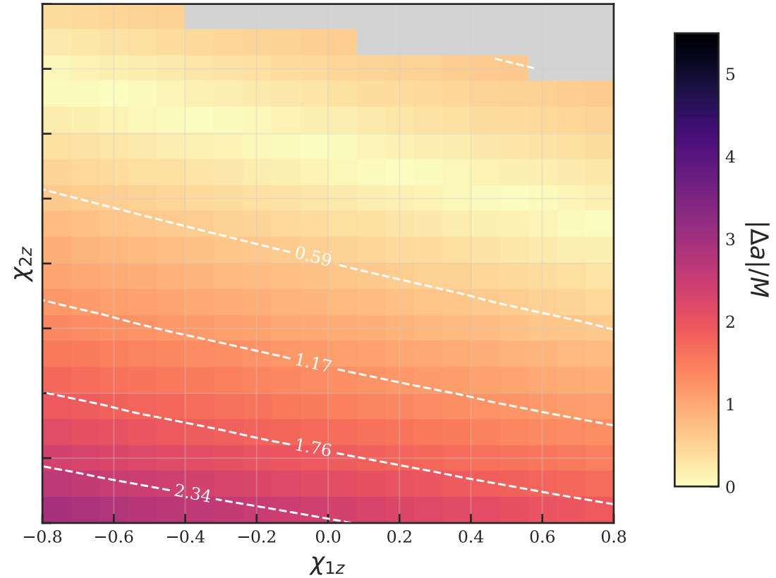
Padé 2PN
