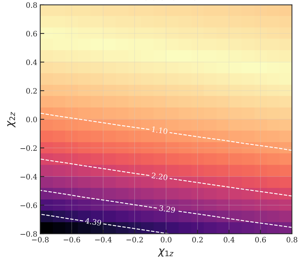
Padé 0PN
