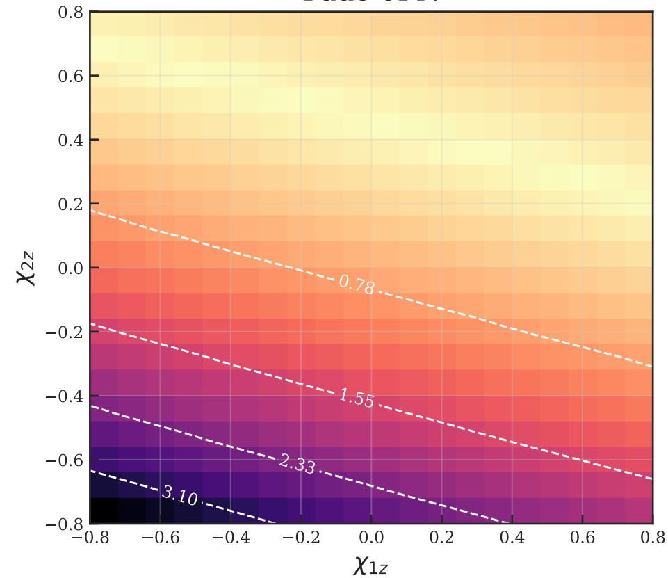
Padé 0PN
