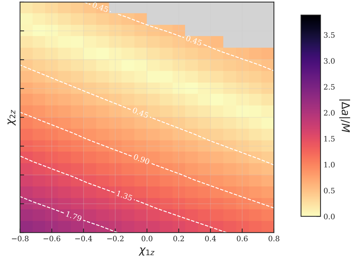
Padé 2PN
