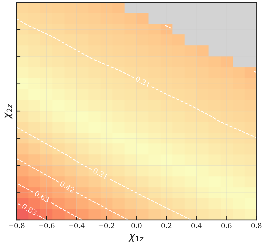
Padé 1PN
