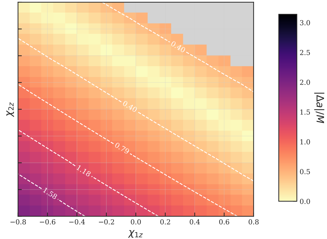
Padé 2PN
