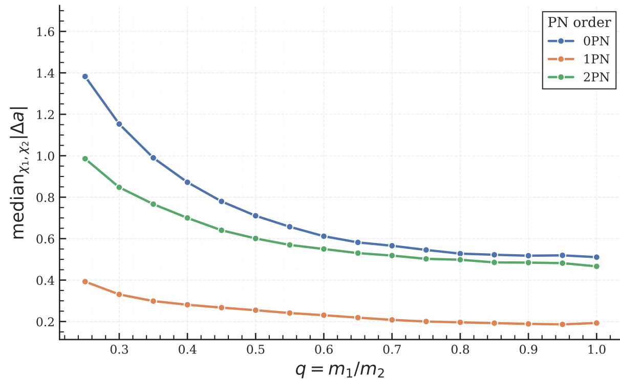
Padé
