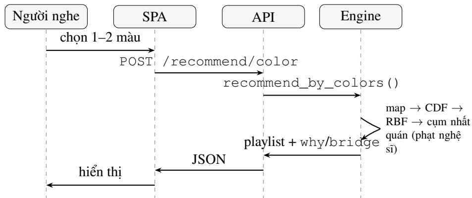
Hình 4.10: Sơ đồ tuần tự UC02 — gợi ý theo màu
