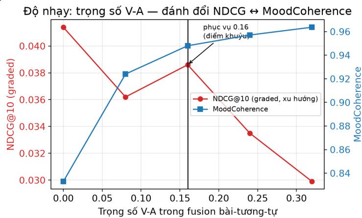
Hình 4.24: Đánh đổi NDCG ↔ MoodCoherence theo trọng số V-A: giá trị phục vụ 0.16 là điểm khuỷu — gần như toàn bộ lợi ích nhất quán cảm xúc đạt được với chi phí NDCG nhỏ
