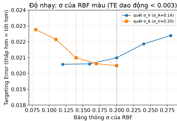
Hình 4.23: Độ nhạy của bảng thông \sigma (RBF màu): TE gần như phẳng trên toàn lưới quét, xác nhận hệ bền với lựa chọn \sigma
