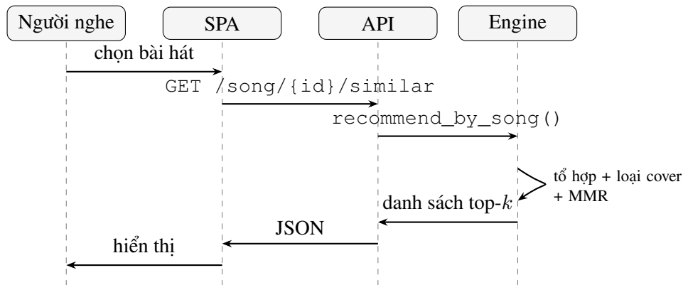
Hình 4.9: Sơ đồ tuần tự UC01 — gợi ý bài tương tự
