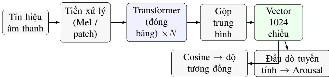
Hình 3.4: Sơ đồ khối sử dụng mô hình học tự giám sát âm nhạc: từ tín hiệu âm thanh tới vector biểu diễn 1024 chiều, dùng cho đo tương đồng và làm đặc trưng cho đầu dò cảm xúc
