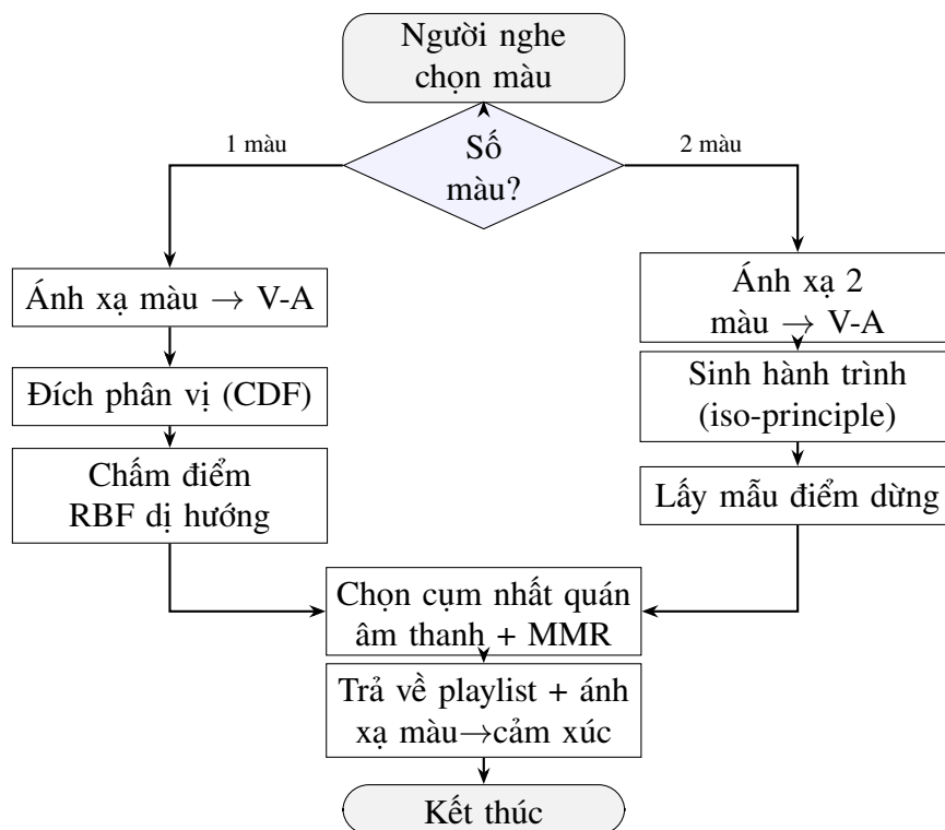
Hình 2.3: Biểu đồ hoạt động của UC02 — gợi ý theo màu (rẽ nhánh một màu / hai màu)
