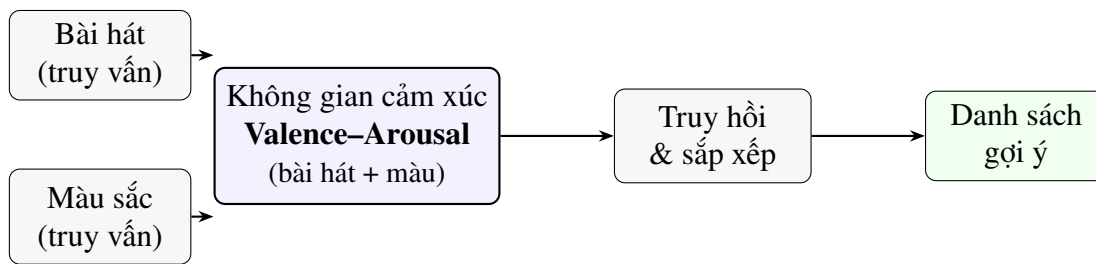
Hình 1.1: Sơ đồ ý tưởng tổng quát của Brightify: bài hát và màu sắc được quy về cùng không gian cảm xúc Valence–Arousal, rồi truy hồi và sắp xếp thành danh sách gợi ý
