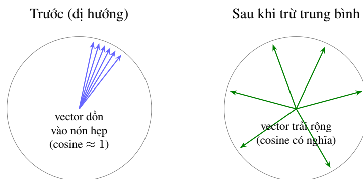
Hình 3.8: Hiện tượng dị hướng và hiệu ứng trừ trung bình: trước khi trừ, các vector dồn vào một nón hẹp nên cosine gần như bằng nhau; sau khi trừ trung bình, chúng trải rộng và cosine khôi phục khả năng phân biệt
