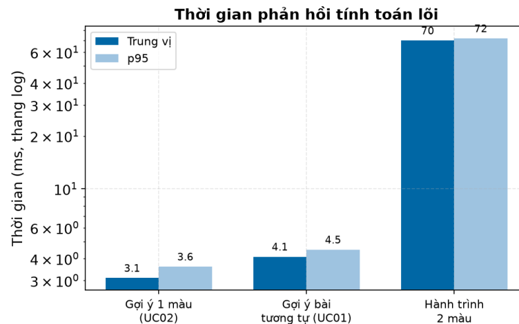
Hình 4.25: Thời gian phản hồi tính toán lỗi theo thao tác (thang log); truy vấn đơn ở mức vài mili-giây
