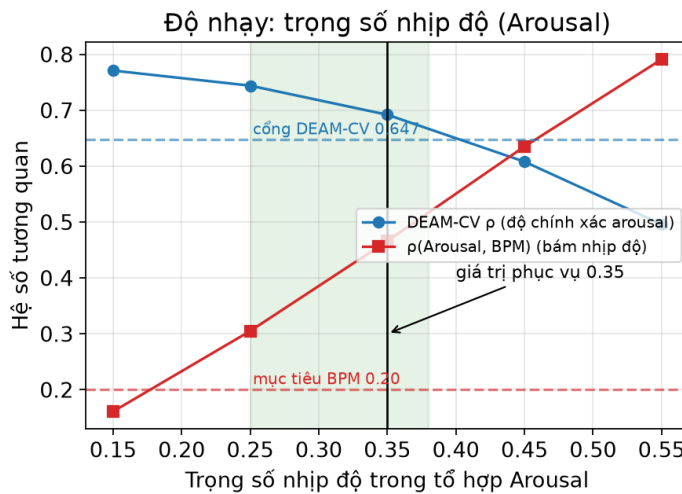
Hình 4.22: Độ nhạy của trọng số nhịp độ: vùng xanh là cửa sổ hợp lệ ( \text{DEAM-CV} \geq 0.647 và \rho(A, \text{BPM}) \geq 0.20 ); giá trị phục vụ 0.35 nằm trong vùng này
