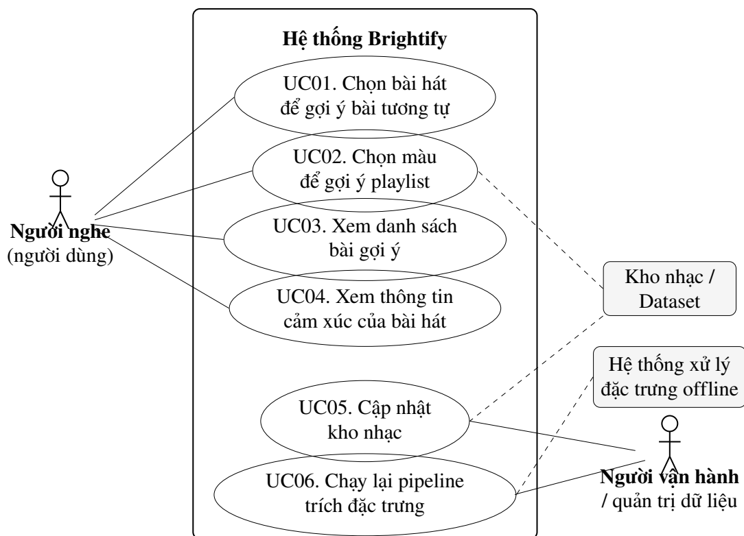
Hình 2.2: Biểu đồ use case tổng quát của hệ thống Brightify
