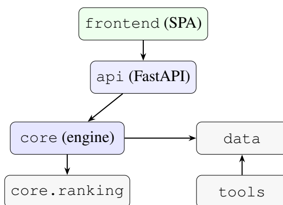
Hình 4.4: Sơ đồ gói: phụ thuộc một chiều giữa các thành phần mã nguồn
