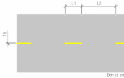
Hình G.1 - Vạch 1.1
