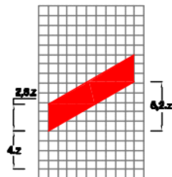
Biển số W.243a: Nơi đường sắt giao không vuông góc với đường bộ
