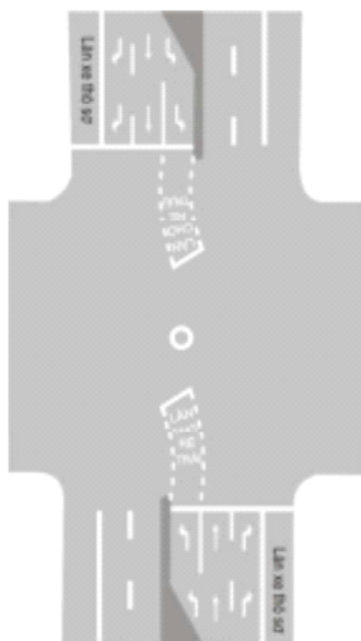
Hình G.42 - Minh họa bố trí vạch 5.3
