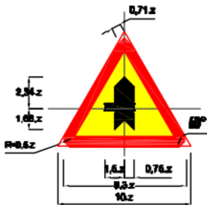
Biển số W.207d: Giao nhau với đường không ưu tiên
