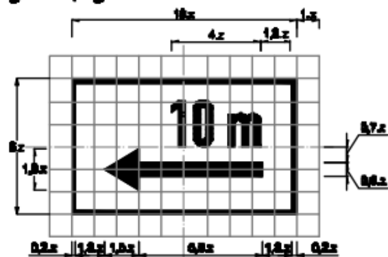
Biển 8.1.3a: Hướng tác dụng của biển
