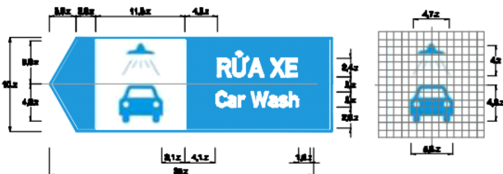
Biển số I.444l: Biển báo chỉ dẫn địa điểm
