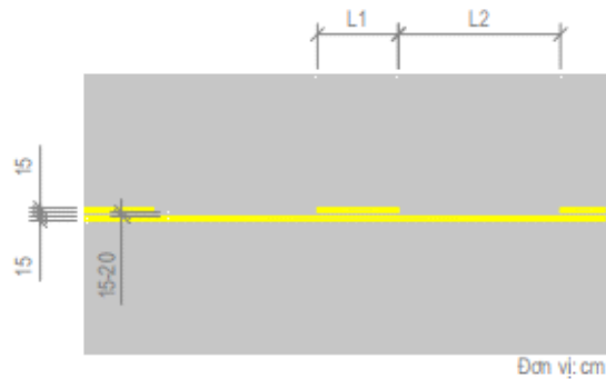
Hình G.4 - Vạch 1.4
