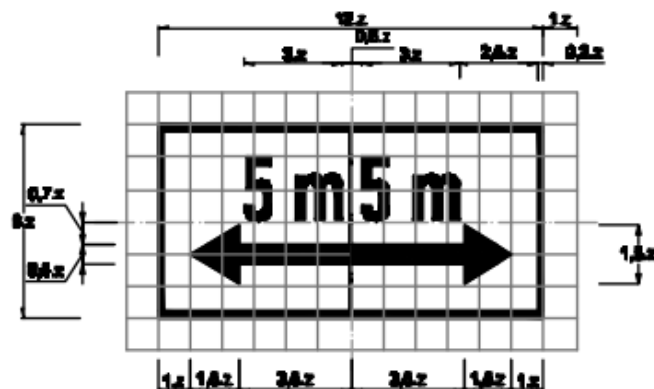
Biển SH.3b : Hướng tác dụng của biển
