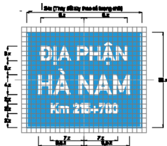
Biển số I.419b: Chỉ dẫn địa giới trên tuyến đường đối ngoại
