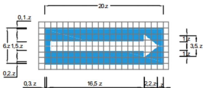
Biển số I.407c: Đường một chiều
