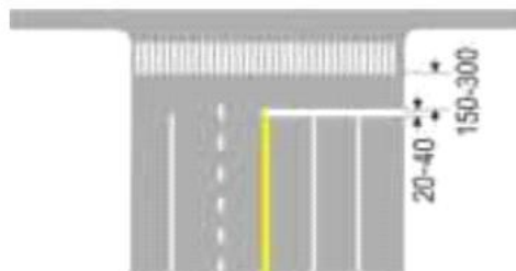
Hình G.46 - Bố trí vạch dừng xe ở nút giao thông có đèn tín hiệu
