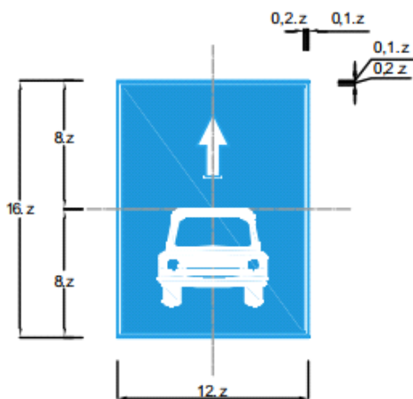
Biển số R.412f: Làn đường dành cho ô tô
