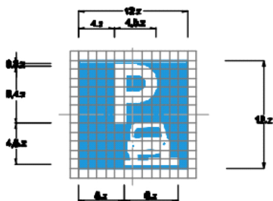
Biển số I.408a: Nơi đỗ xe một phần trên hè phố
