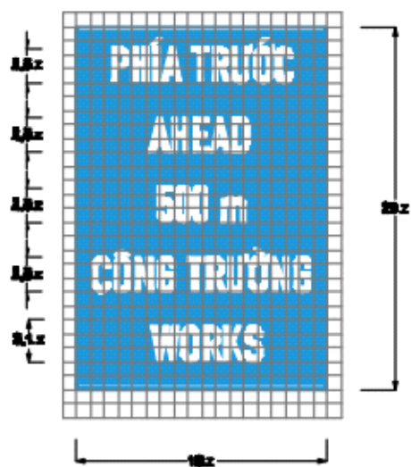
Biển số I.441b: Báo hiệu phía trước có công trình thi công
