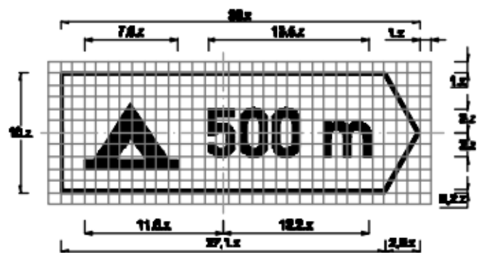
Biển số 2.G.7 : Biển chỉ dẫn tới địa điểm cắm trại, tới nhà trọ
