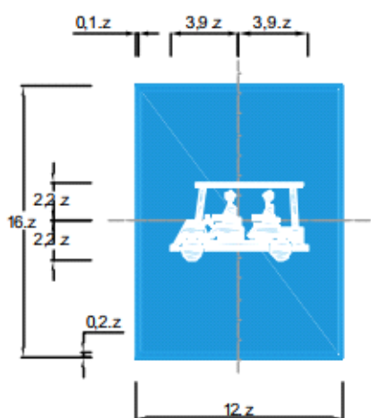
Biển số R.403h: Đường dành cho xe chở người bốn bánh gắn động cơ
