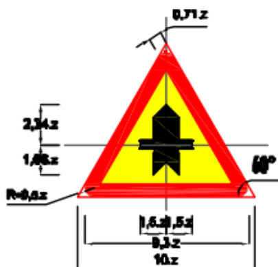
Biển số W.207b: Giao nhau với đường không ưu tiên
