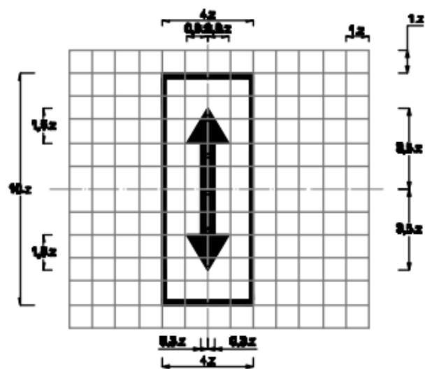
Biển số 8.503f: Hướng tác dụng của biển
