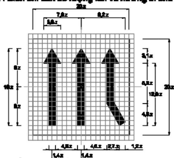
Biển số 8.G.11c: Biển chỉ dẫn số lượng làn và hướng đi cho từng làn
