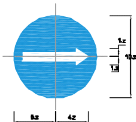
Biển số R.301b: Các xe chỉ được rẽ phải
