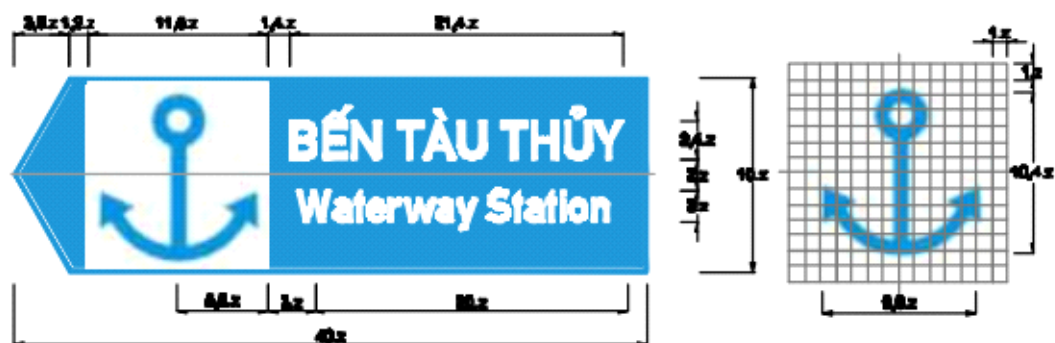
Biển số I.444f: Biển báo chỉ dẫn địa điểm
