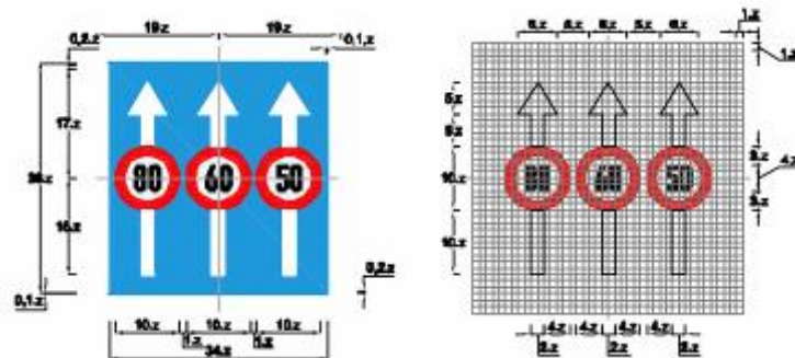
Biển số P.127b: Biển gộp tốc độ tối đa cho phép theo làn đường đặt bên đường hoặc trên cột cần vượn
