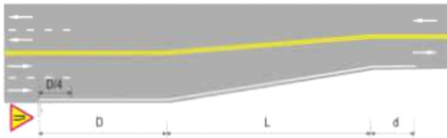
Hình G.21 - Bố trí vạch sơn khu vực chuyển tiếp giữa đường 4 làn xe và đường 2 làn xe
