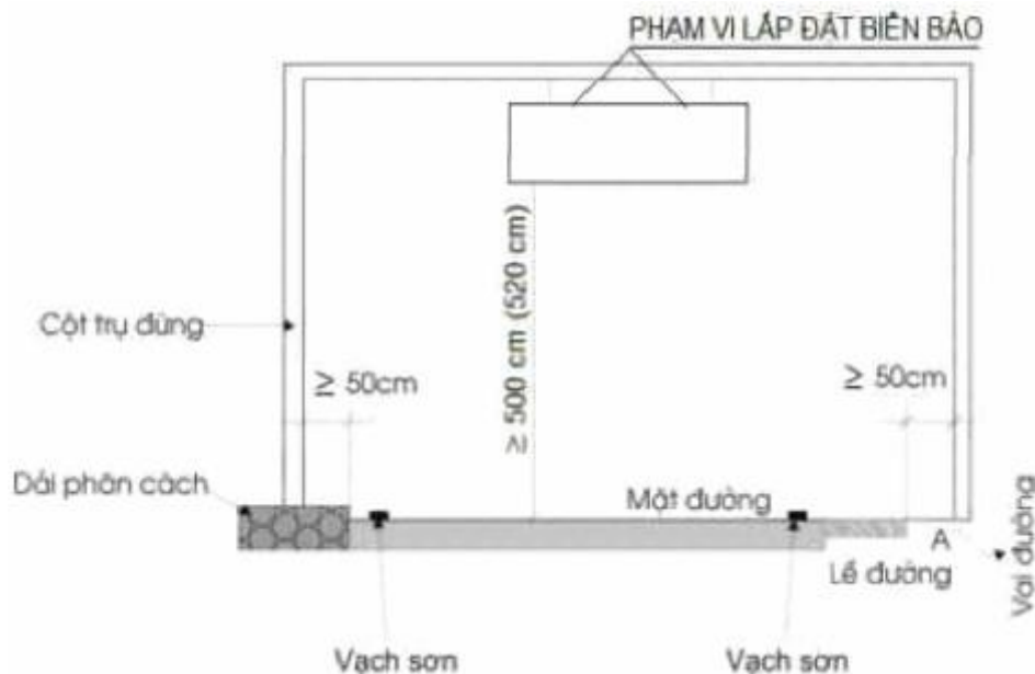
Hình 2 - Giá long môn
