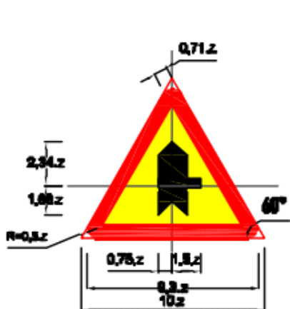
Biển số W.207b: Giao nhau với đường không ưu tiên
