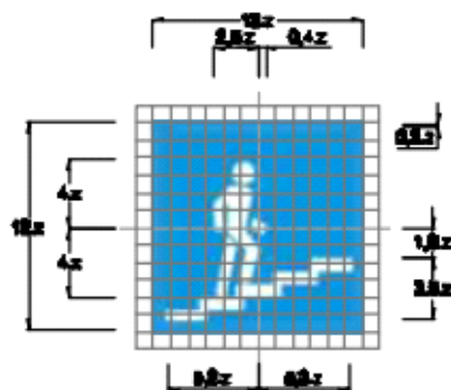
Biển số I.424b: Cầu vượt qua đường cho người đi bộ
