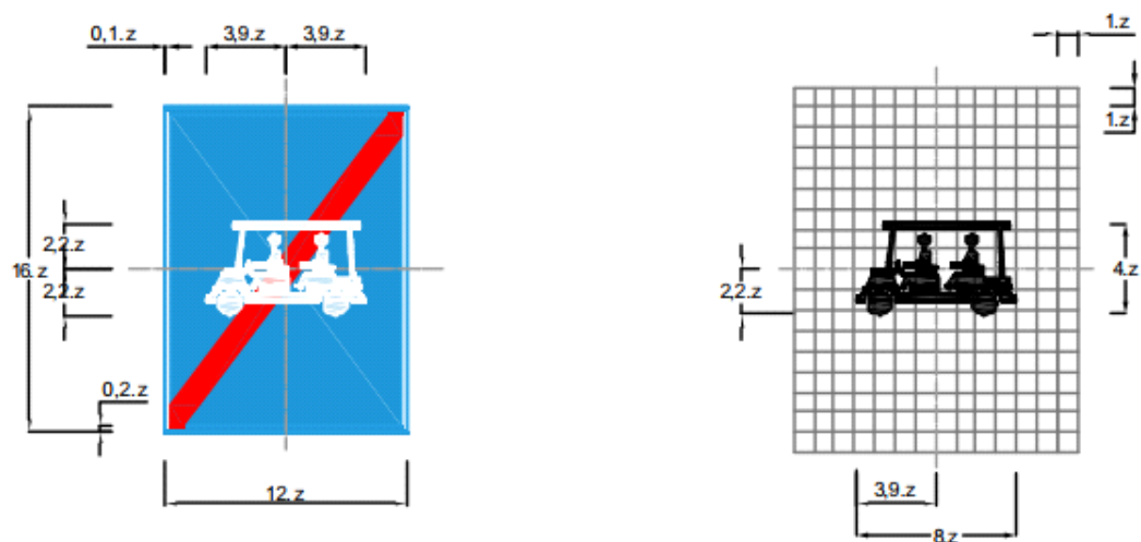
Biển số R.404k: Hết đoạn đường dành cho xe chở hàng, xe chở người bốn bánh gắn động cơ
