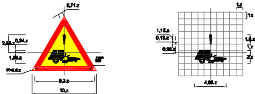
Biển số W.245a: Đi chậm
