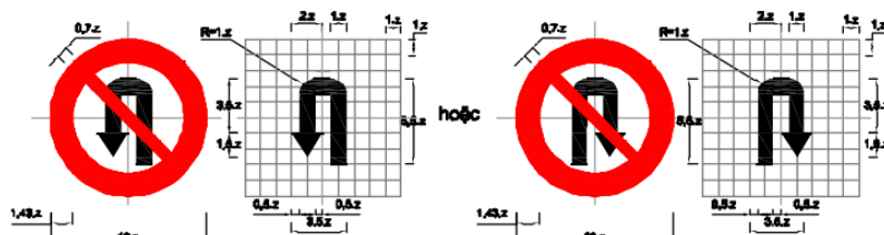
Biển số P.124a: Cấm quay đầu xe
