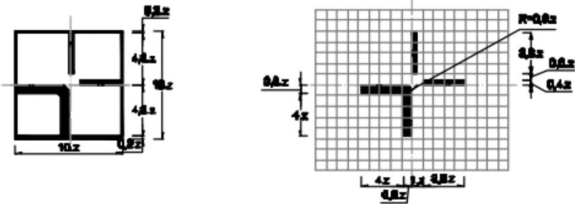
Bản số 3.566a : Hướng đường ưu tiên
