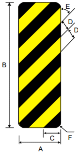
Biển số IE.468a
