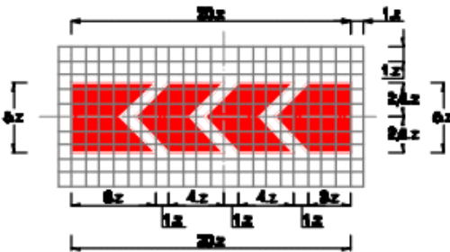
Bản số 3.567 : Hướng rẽ
