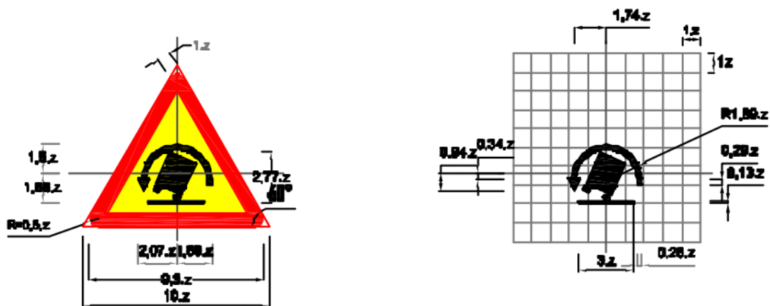
Biển số W.201c: Chỗ ngoặt nguy hiểm có nguy cơ lật xe bên phải khi đường cong vòng sang trái
