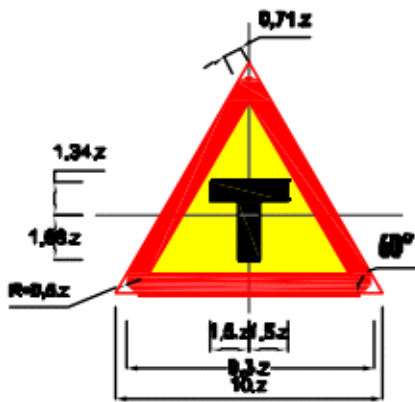
Biển số W.205e: Đường giao nhau
