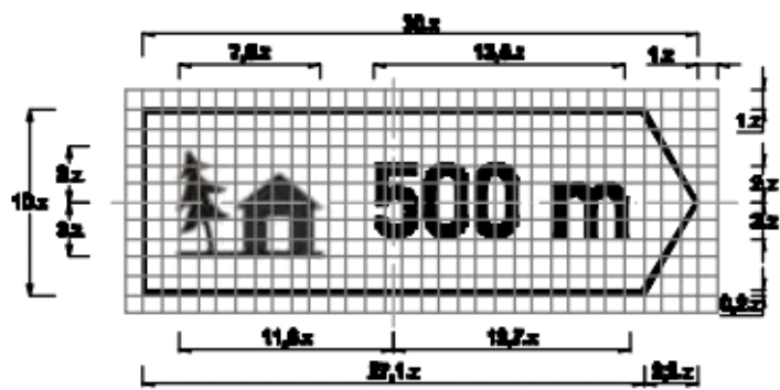
Biển số 2.G.8: Biển chỉ dẫn tới địa điểm cắm trại, tới nhà trọ
