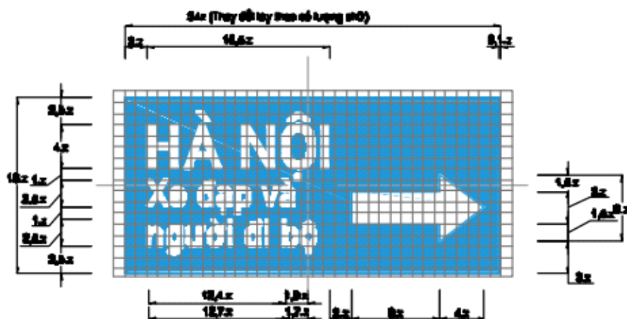
Biển số I.417c: Chỉ hướng đường phải đi cho từng loại xe
