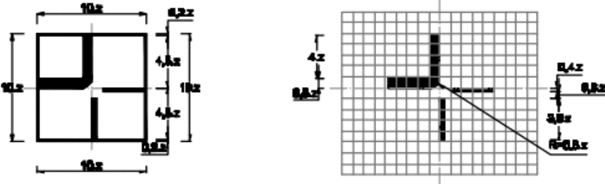
Bản số 3.566b : Hướng đường ưu tiên
