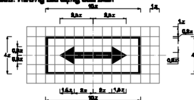
Bản số 3.503c: Hướng tác dụng của biển
