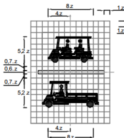
Biển số R.403k: Đường dành cho xe chở hàng, xe chở người bốn bánh gắn động cơ
