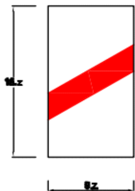
Biển số W.243b: Nơi đường sắt giao không vuông góc với đường bộ
