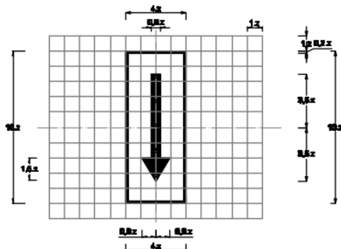
Bản số 3.503d: Hướng tác dụng của biển
