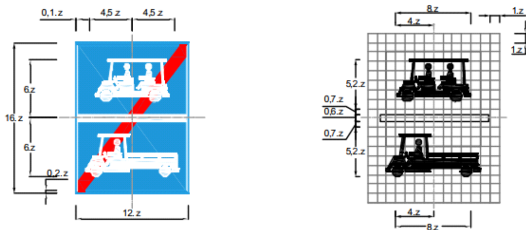
Biển số R.404k: Hết đoạn đường dành cho xe chở hàng, xe chở người bốn bánh gắn động cơ
