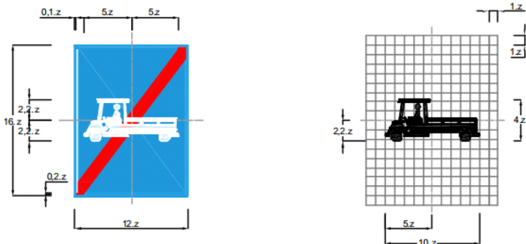
Biển số R.404h: Hết đoạn đường dành cho xe chở người bốn bánh gắn động cơ
