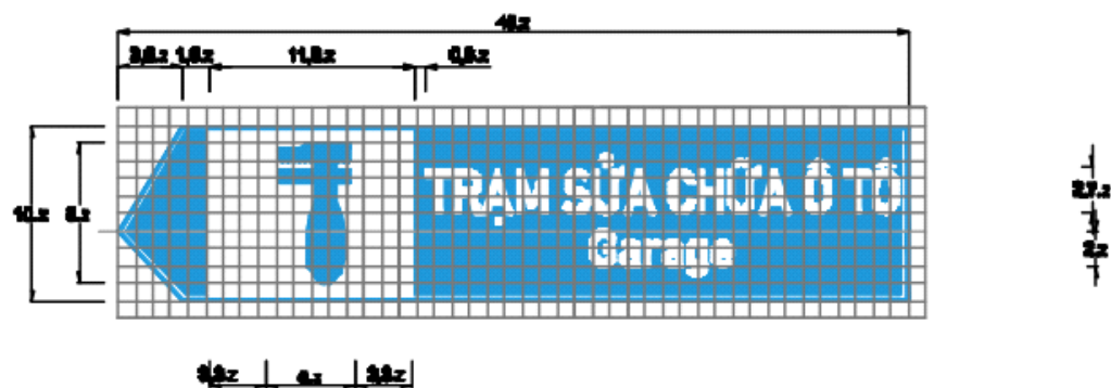
Biển số I.445a: Biển báo mô tả tình trạng đường
