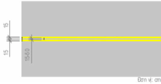
Hình G.3 - Vạch 1.3
