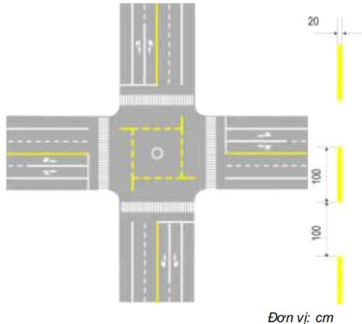
Hình G.54 - Vạch xác định khu vực cấm xe thô sơ trong nút giao
