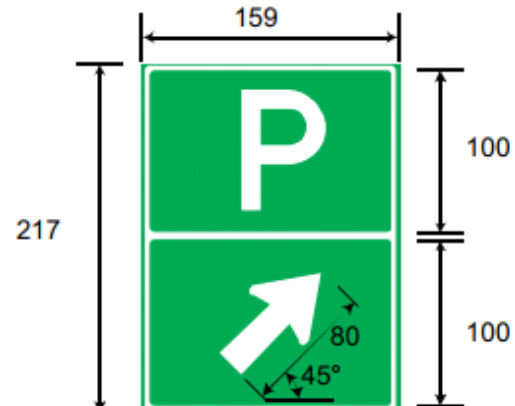
b) Biển số IE.457b
