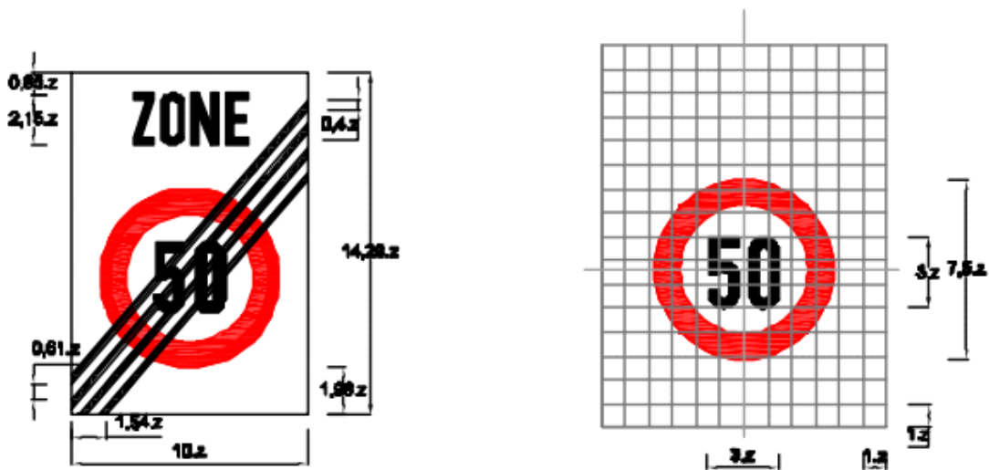
Biển số R.E,10d: Hết hạn chế tốc độ tối đa trong khu vực
