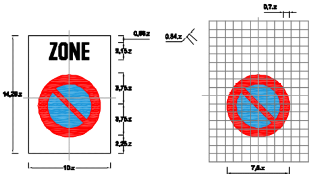
Biển số R.E.9b: Cấm đỗ xe trong khu vực
