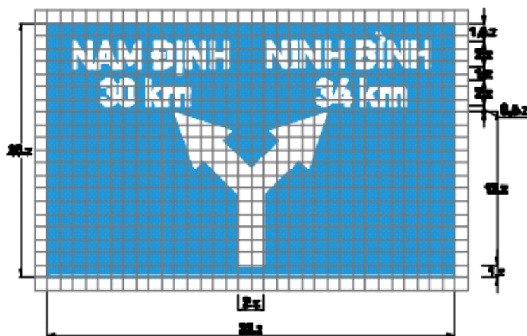
Biển số I.414b: Chỉ hướng đường
