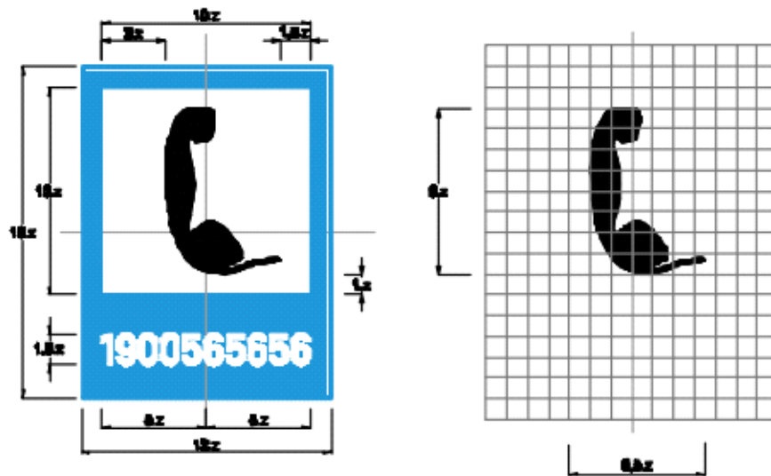
Biển số I.430: Điện thoại
