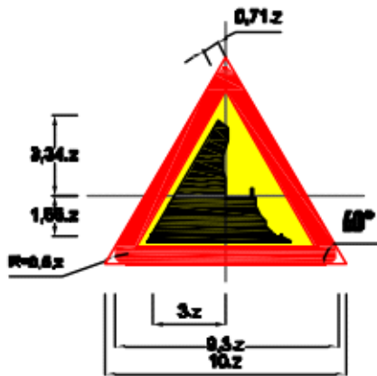
Biển số W.223b: Vách núi nguy hiểm
