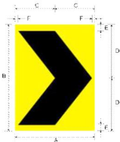
Biển số IE.469
