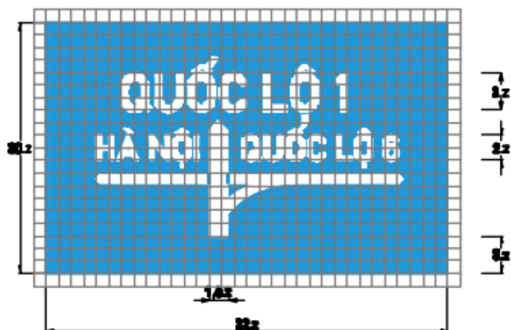
Biển số I.1447b: Biển báo cầu vượt liên thông
