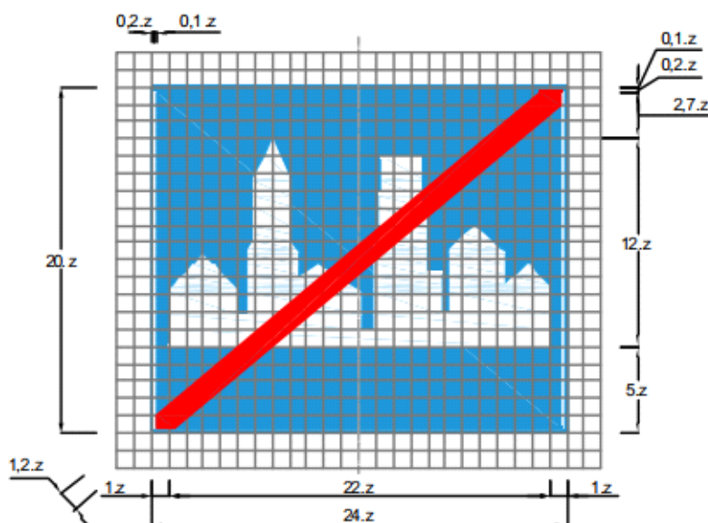
Biển số R.420: Hết khu đông dân cư
