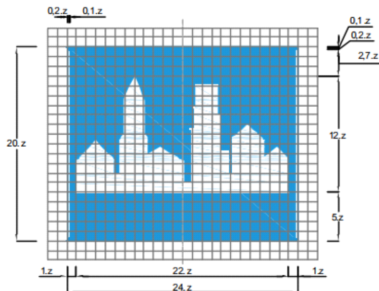
Biển số R.420: Hết khu đông dân cư
