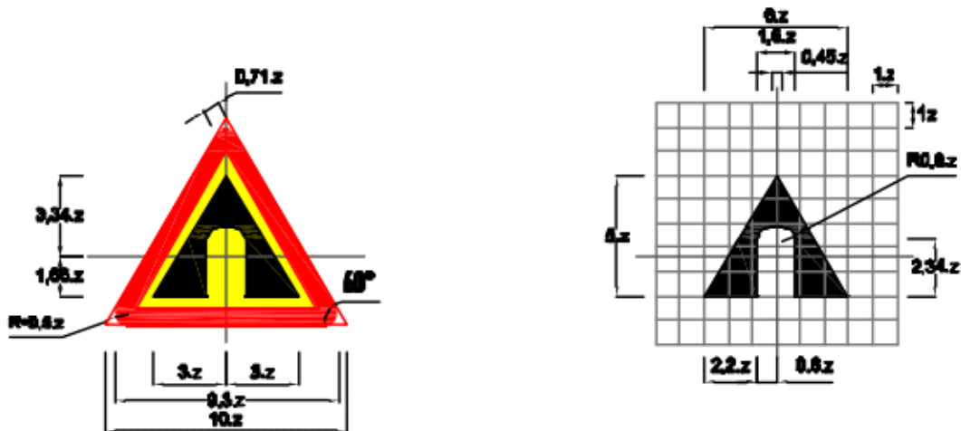
Biển số W.218: Cửa chui
