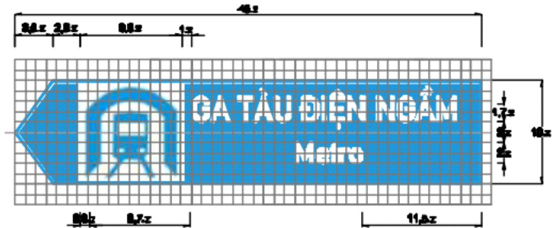
Biển số L444l: Biển báo chỉ dẫn địa điểm
