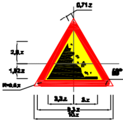
Biển số W.228b: Đá lở
