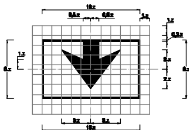
Biển số 3.504 : Làn đường
