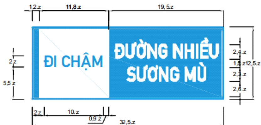
Biển số I.445d: Biển báo mô tả tình trạng đường
