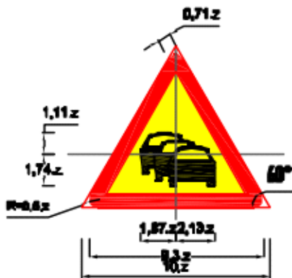
Biển số W.241: Ủy tắc giao thông
