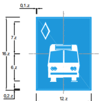
Biển số R.403c: Đường dành cho xe buýt
