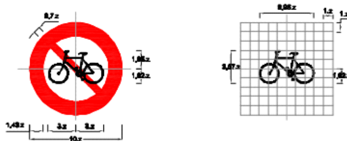
Biển số P.110a: Cấm xe đạp
