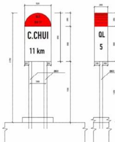
Hình I.1 - Cột kilômét dạng cột thấp
