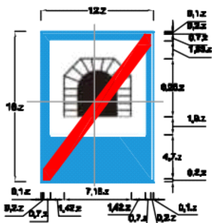
Biển số R. E.11b: Hết đường hầm
