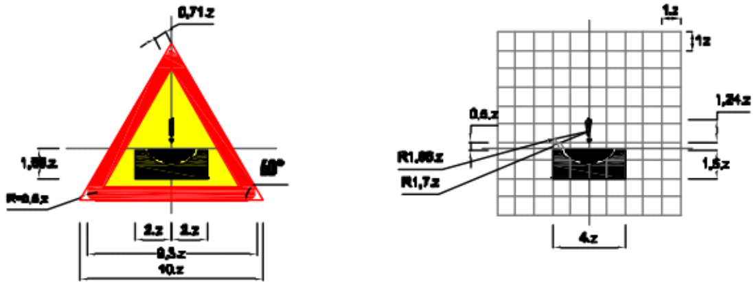
Biển số W.217: Bến phà
