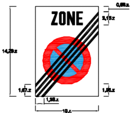
Biển số R.E,10b: Hết cấm đỗ xe theo giờ trong khu vực
