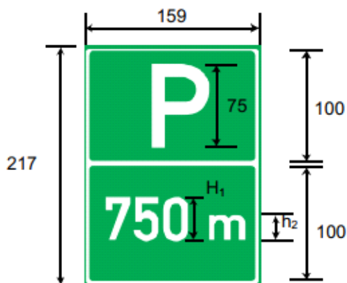
a) Biển số IE.457a
