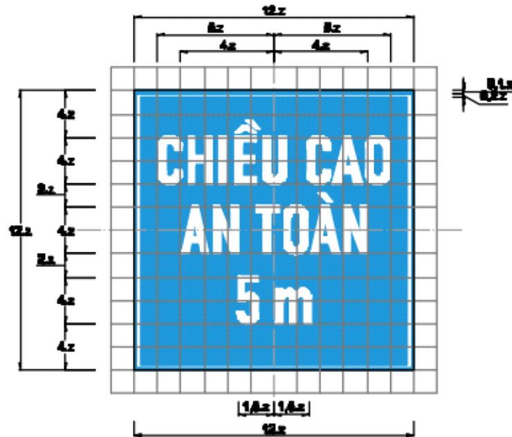
Biển số 8.508b : Thuyết minh biển chính
