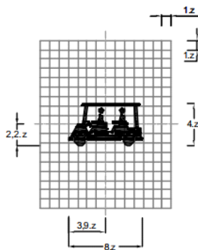
Biển số R.403k: Đường dành cho xe chở hàng, xe chở người bốn bánh gắn động cơ
