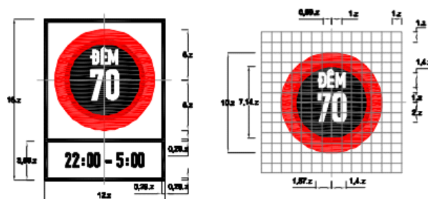
Biển số P.127a: Tốc độ tối đa cho phép về ban đêm
