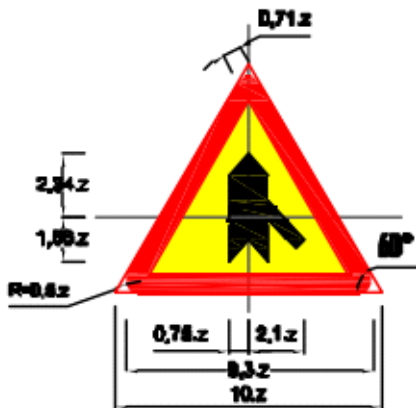
Biển số W.207h: Giao nhau với đường không ưu tiên
