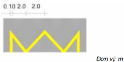
Hình G.72 - Chi tiết vạch số 9.2
