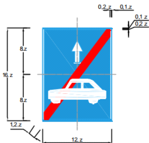
Biển số R.421j: Hết làn đường dành cho xe ô tô con
