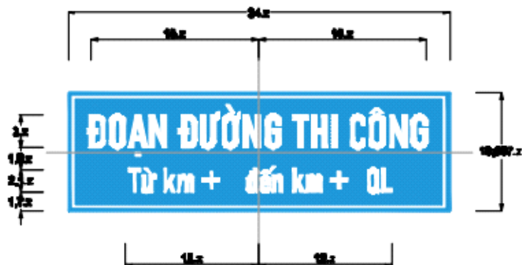
Biển số I.440: Đường đang thi công
