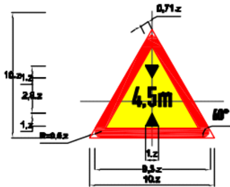
Biển số W.240: Đường hãm
