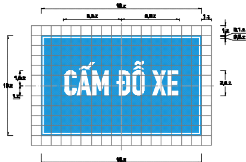
Biển số 8.508b : Thuyết minh biển chính
