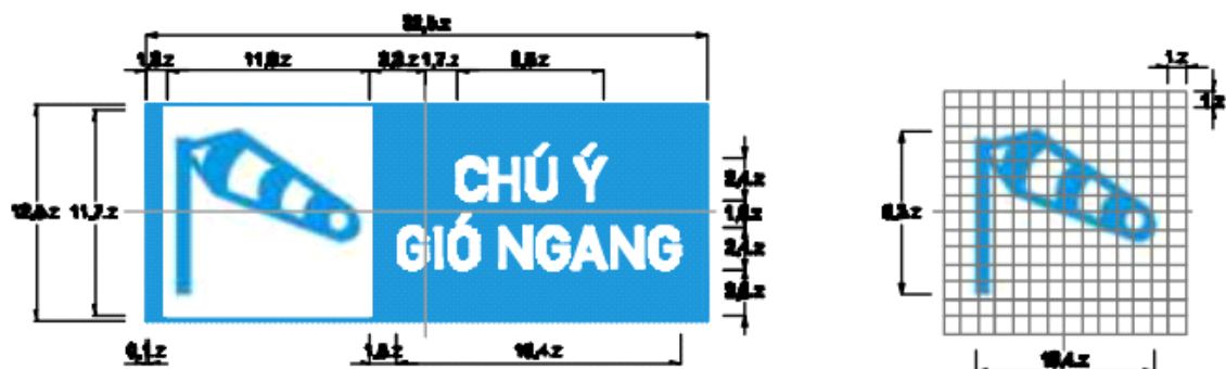
Biển số I.445g: Biển báo mô tả tình trạng đường
