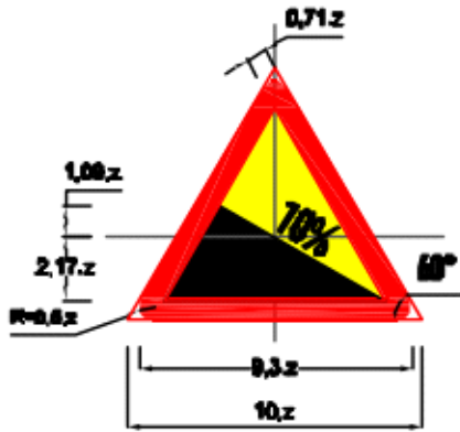
Biển số W.220: Dốc lên nguy hiểm
