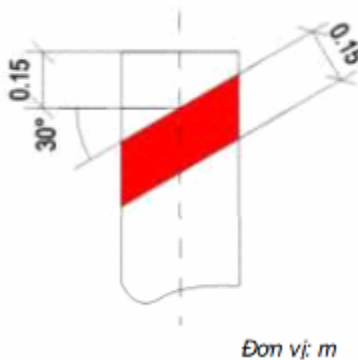
Hình G.67 - Chi tiết vạch 8.4
