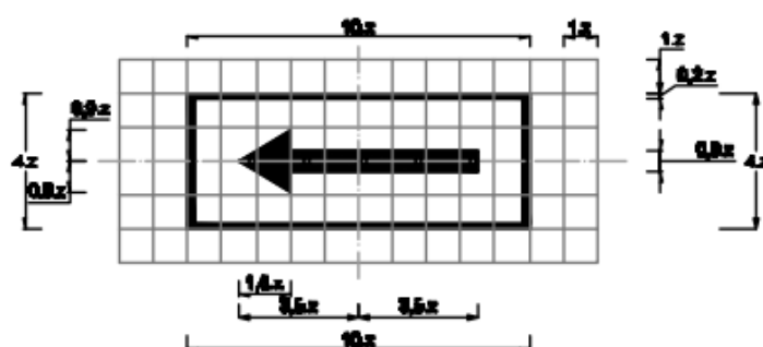
Bản số 3.503d: Hướng tác dụng của biển
