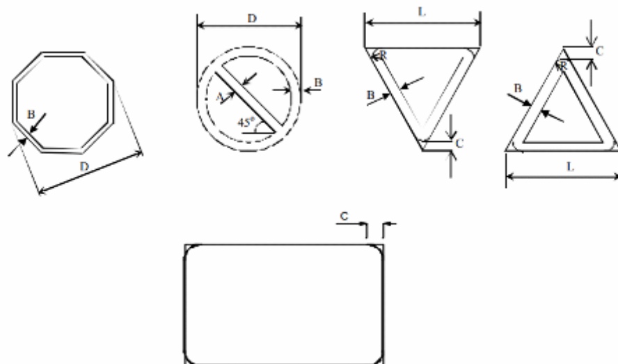
Hình 1 - Kích thước các loại biển báo
