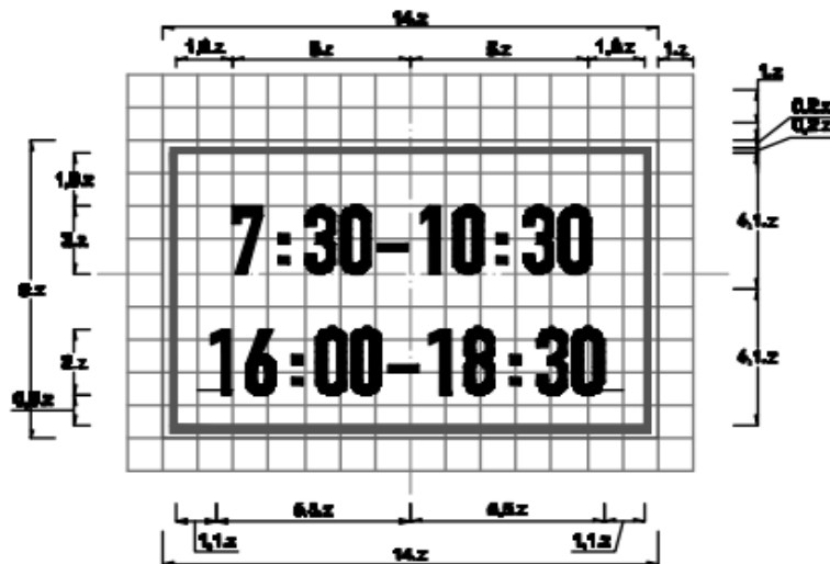
Biển số S.502b : Biểu thị thời gian
