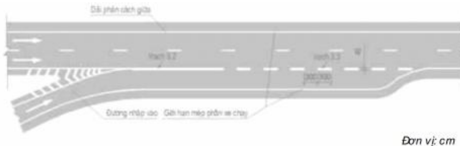
Hình G.17 - Minh họa bố trí vạch sơn khu vực nhập làn kiểu có làn chuyển tiếp song song
