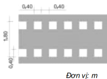
Hình G.53 - Vạch xe đạp qua đường
