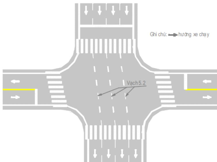
Hình G.41 - Minh họa bố trí vạch 5.2
