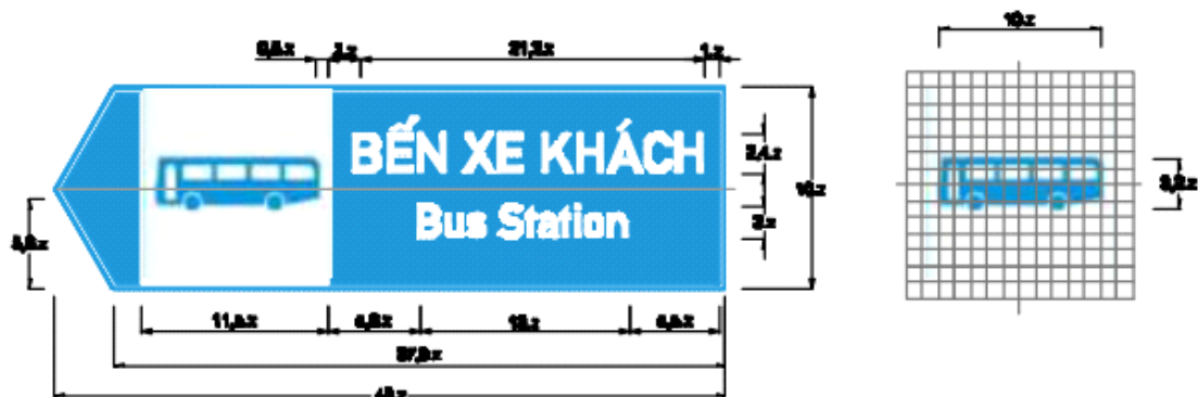
Biển số I.444e: Biển báo chỉ dẫn địa điểm
