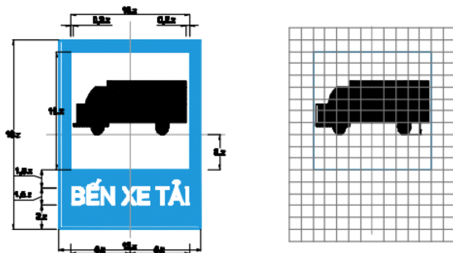
Biển số I.434b: Bến xe tải
