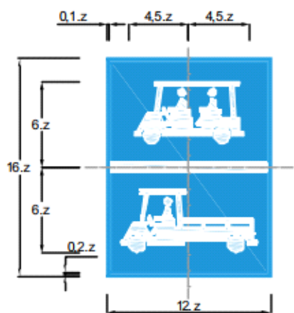
Biển số R.403k: Đường dành cho xe chở hàng, xe chở người bốn bánh gắn động cơ
