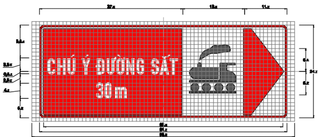
Biển số 3.510b : Chú ý đường sắt
