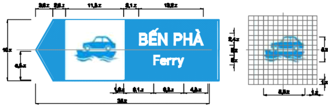
Biển số L444k: Biển báo chỉ dẫn địa điểm
