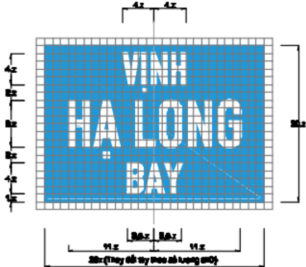
Biển số I.422b: Di tích lịch sử
