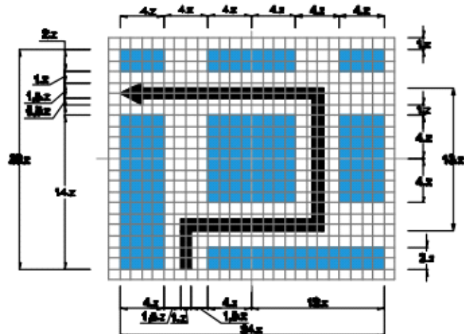
Biển số I.419a: Chỉ dẫn địa giới
