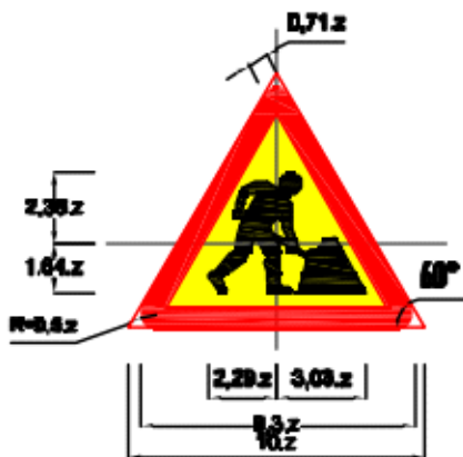
Biển số W.227: Công trường
