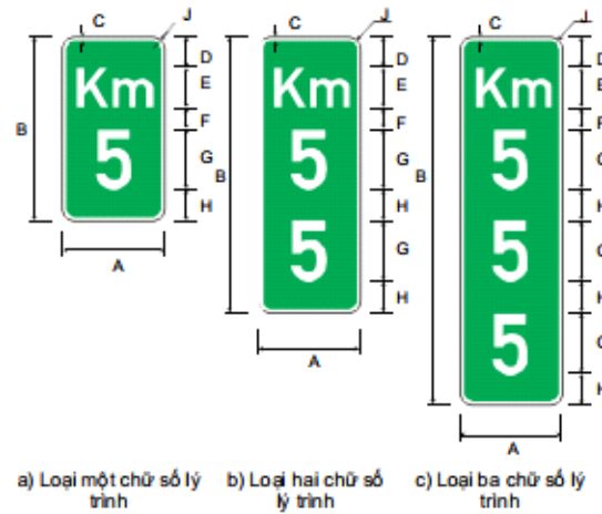
Hình I.2 - Cột kilômét dạng cột cao
