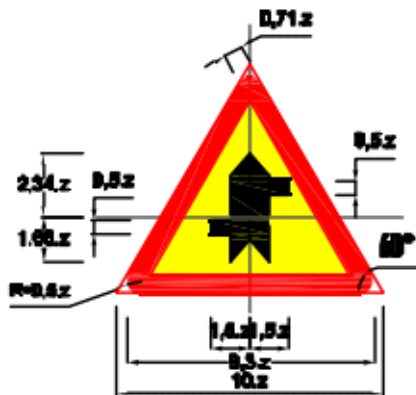
Biển số W.207e: Giao nhau với đường không ưu tiên
