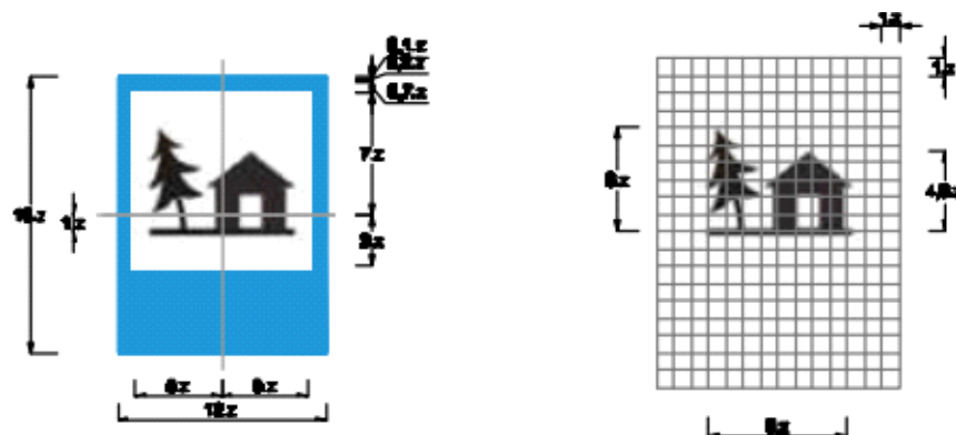
Biển số I.433e: Báo hiệu nhà trọ
