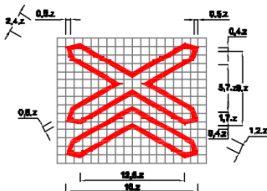
Biển số W.242b: Nơi đường sắt giao vuông góc với đường bộ
