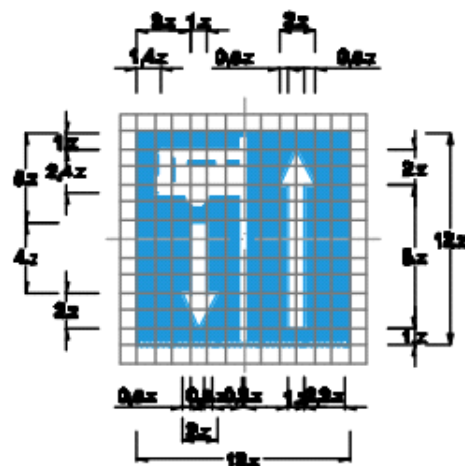
Biển số I.413b: Rẽ ra đường có làn đường dành cho ô tô khách
