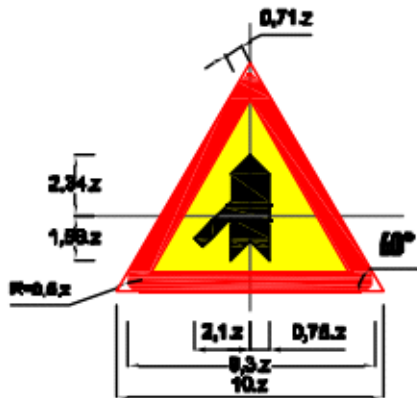
Biển số W.207f: Giao nhau với đường không ưu tiên
