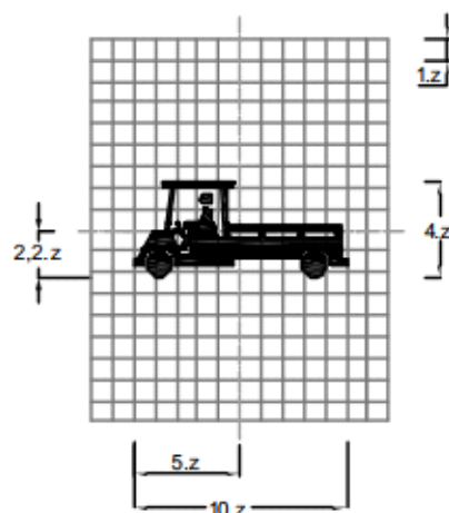
Biển số R.403h: Đường dành cho xe chở người bốn bánh gắn động cơ
