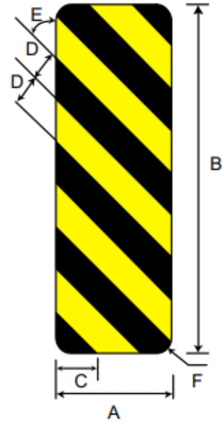
Biển số IE.468c
