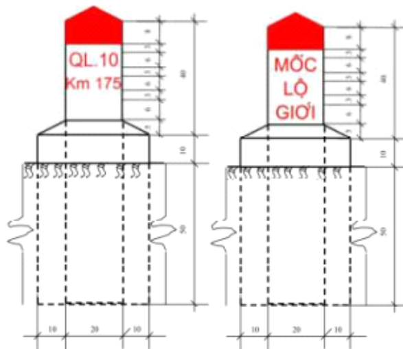
Hình I.4 - Cọc mốc lộ giới
