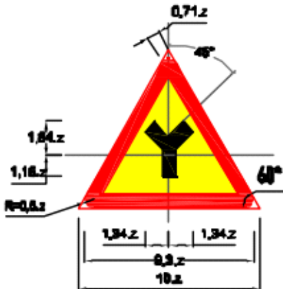
Biển số W.205e: Đường giao nhau
