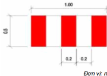
Hình G.65 - Chi tiết vạch 8.2
