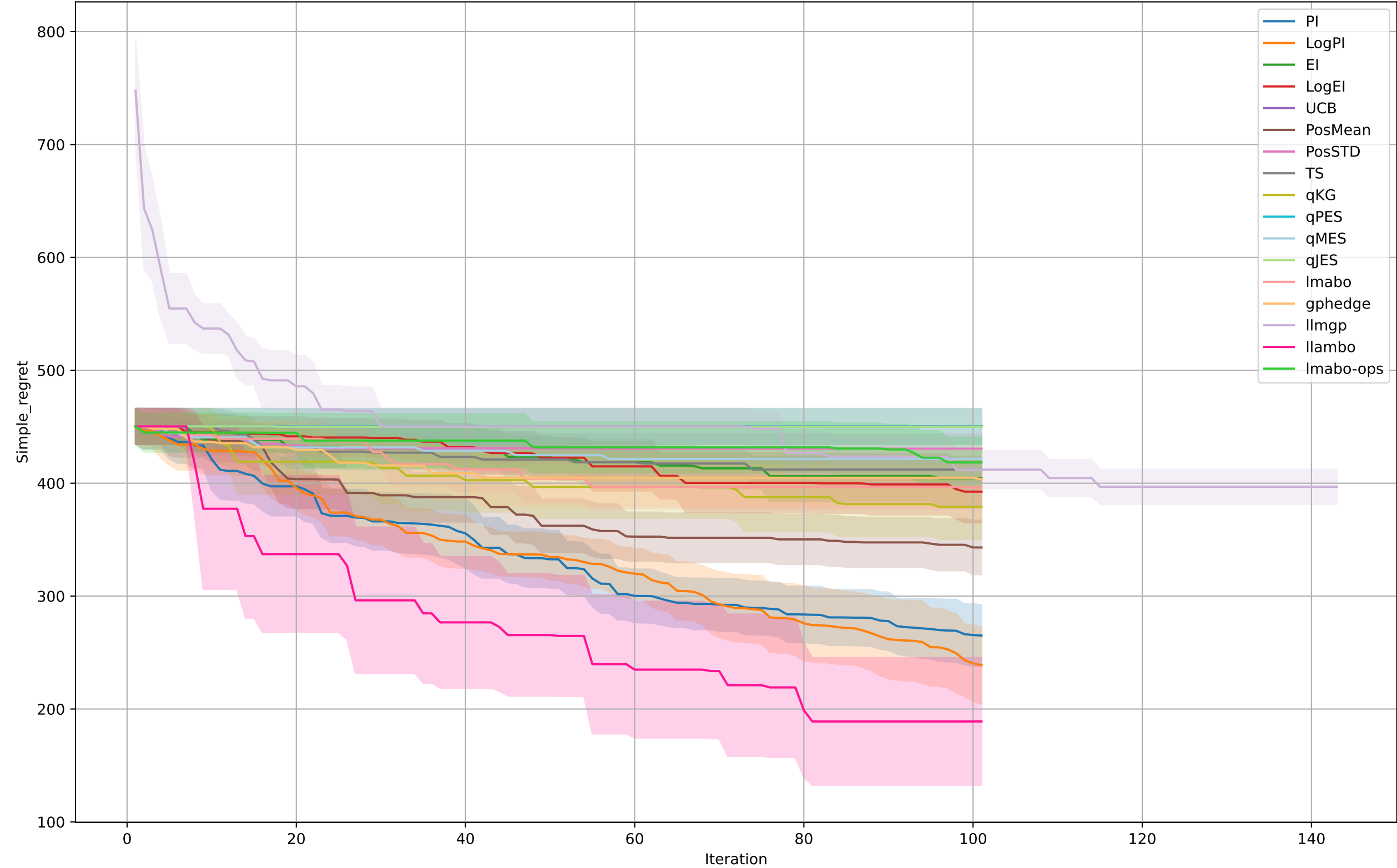
StyblinskiTang
