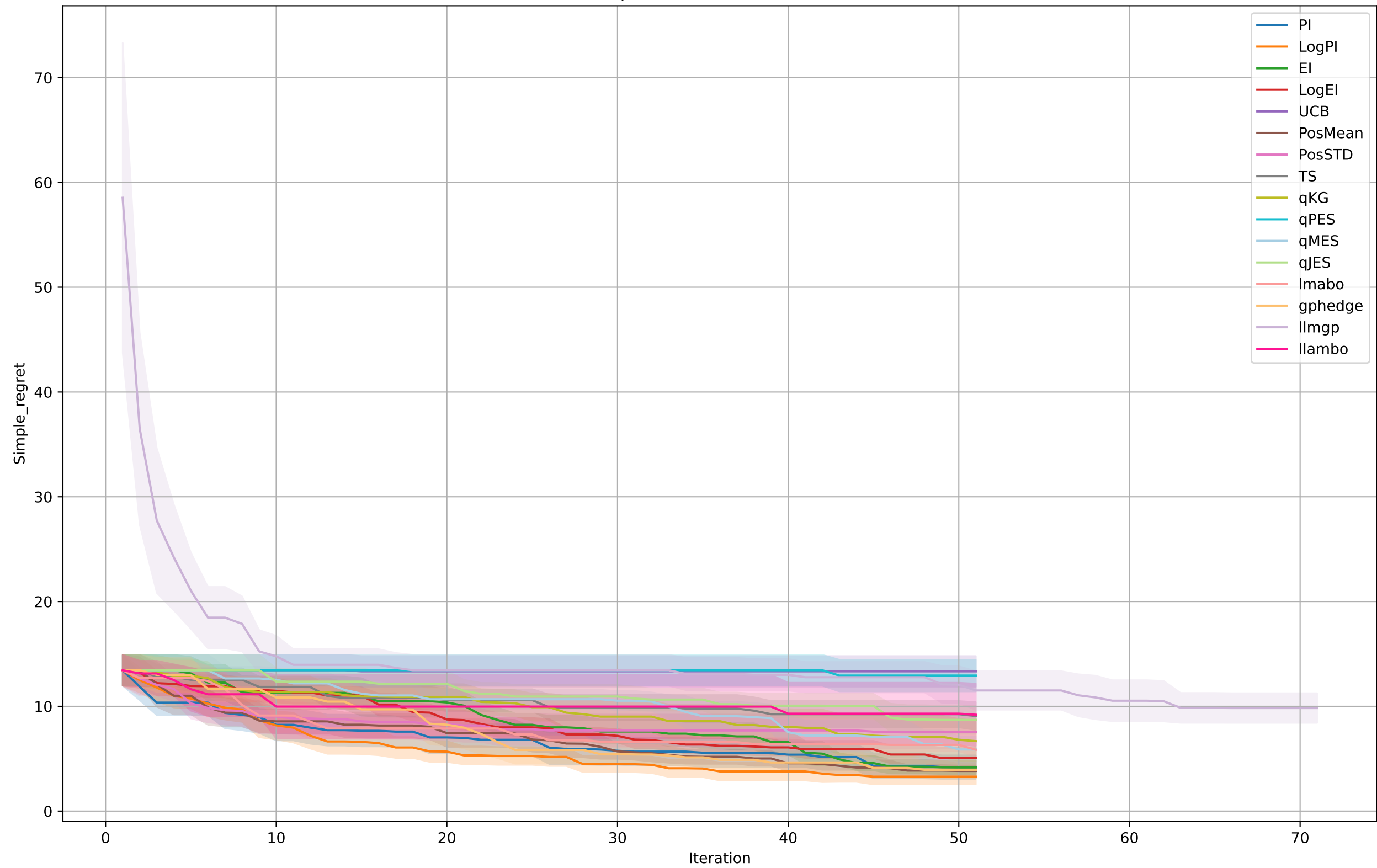
CompositeGriewankRosenbrock
