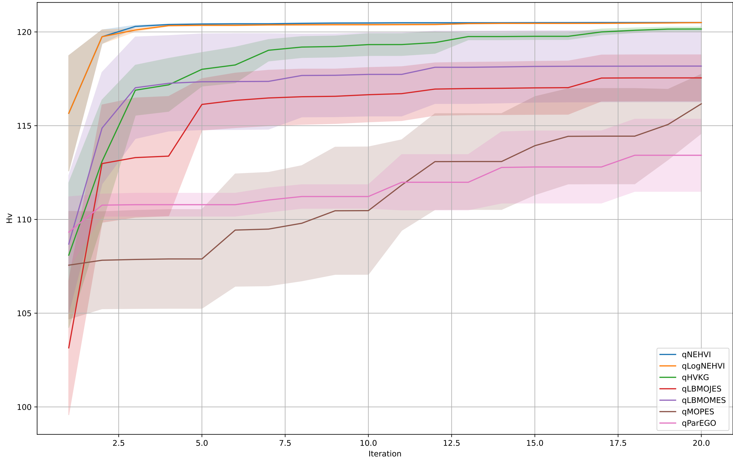
ZDT1
