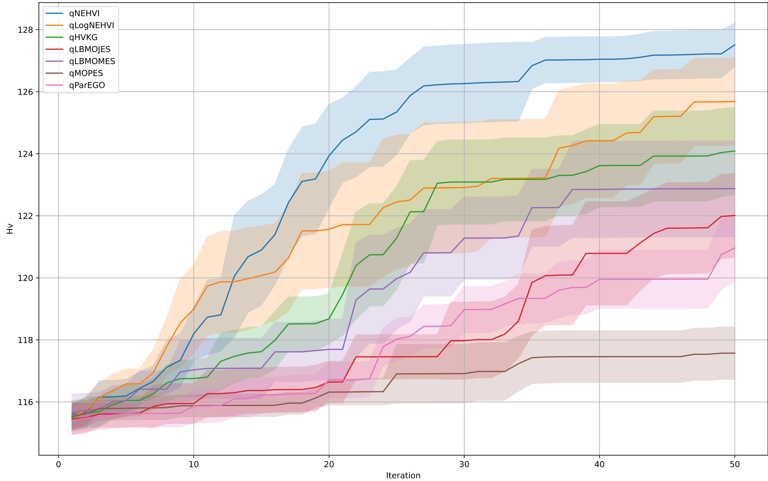
ZDT3
