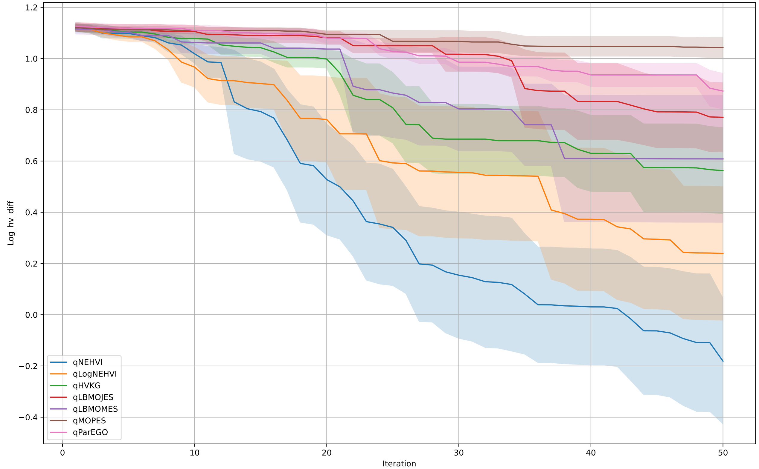
ZDT3
