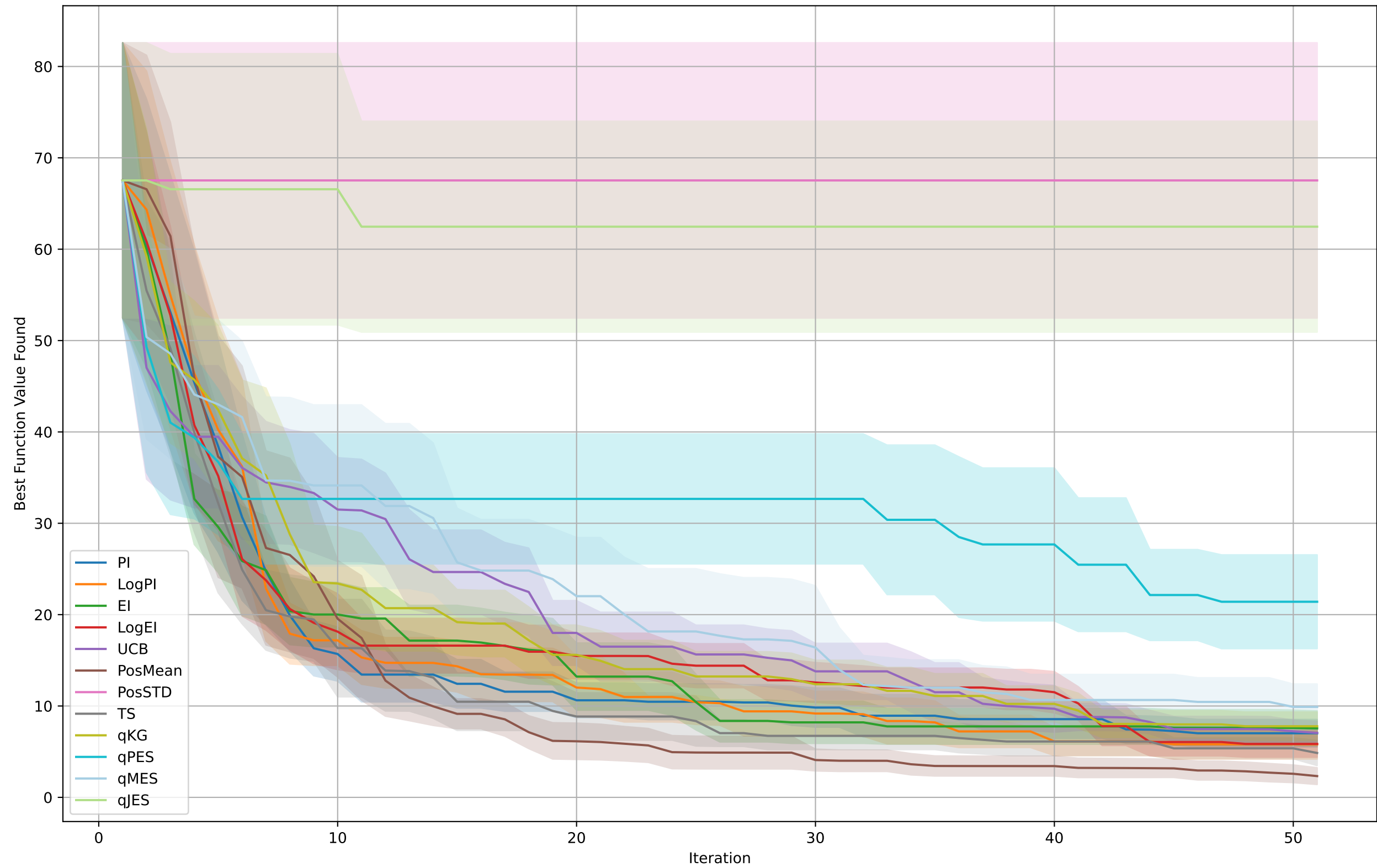
BO on Bukin
