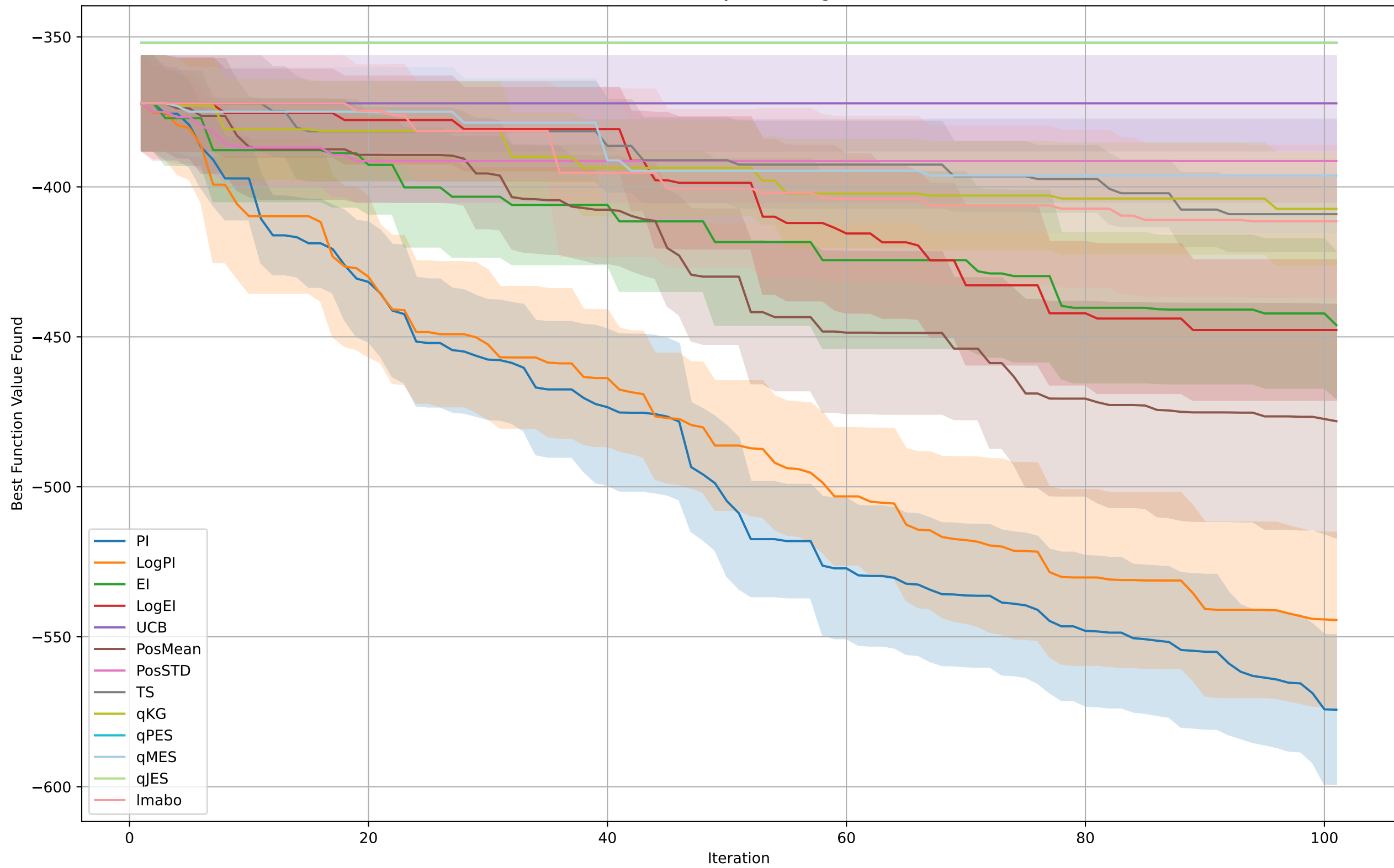
BO on StyblinskiTang
