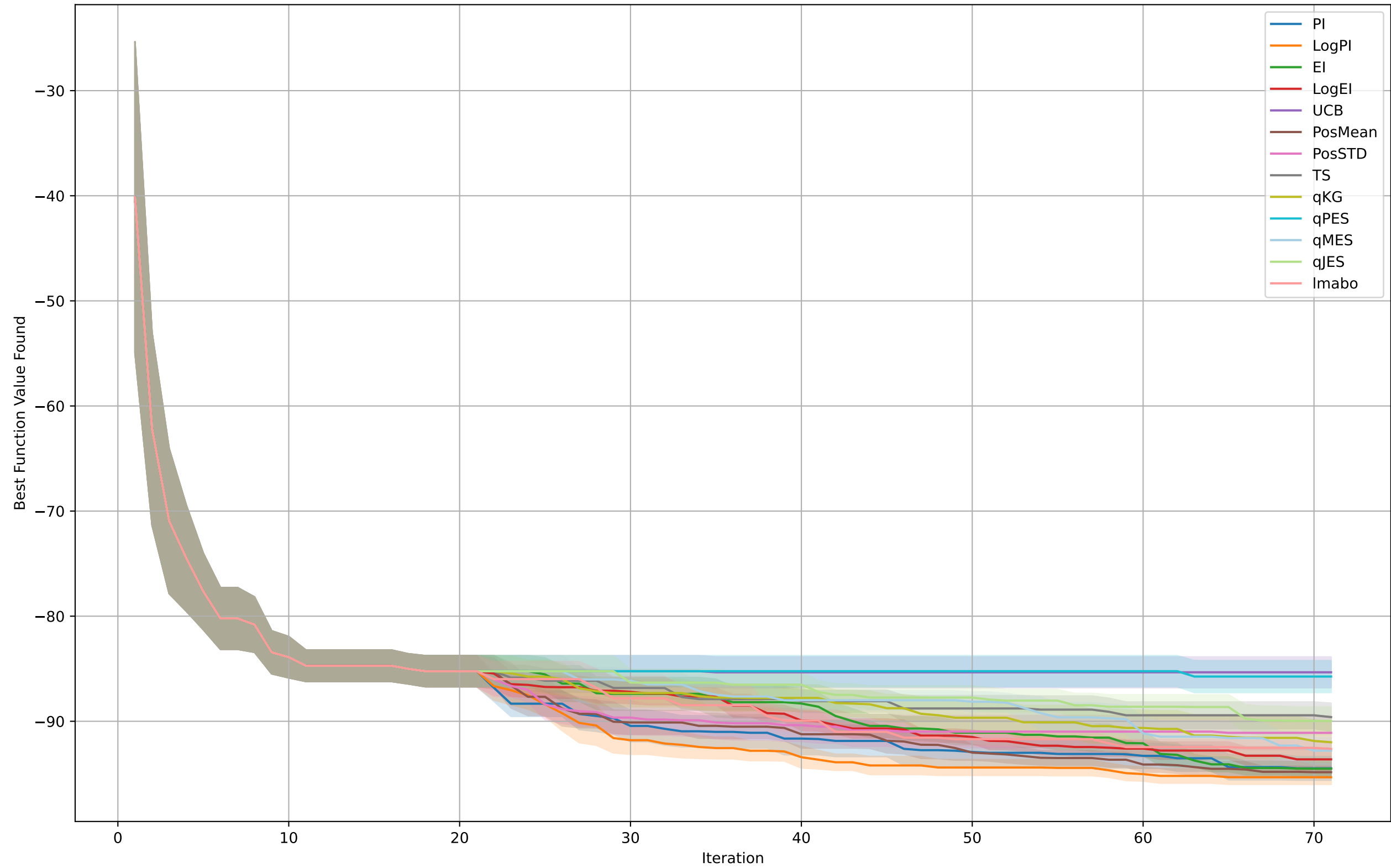
CompositeGriewankRosenbrock
