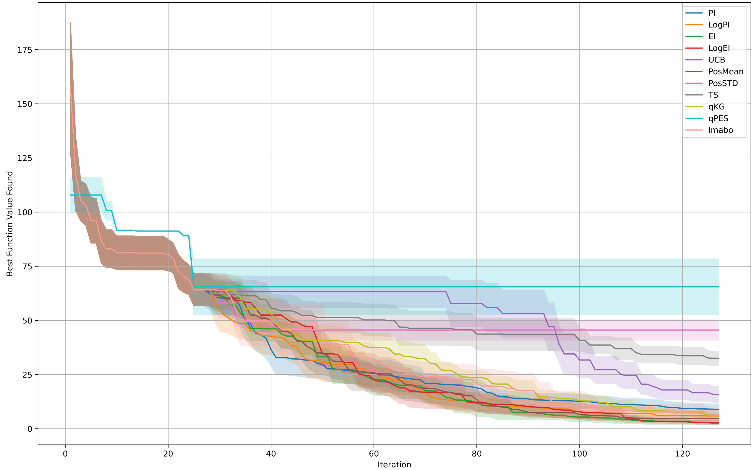
Levy
