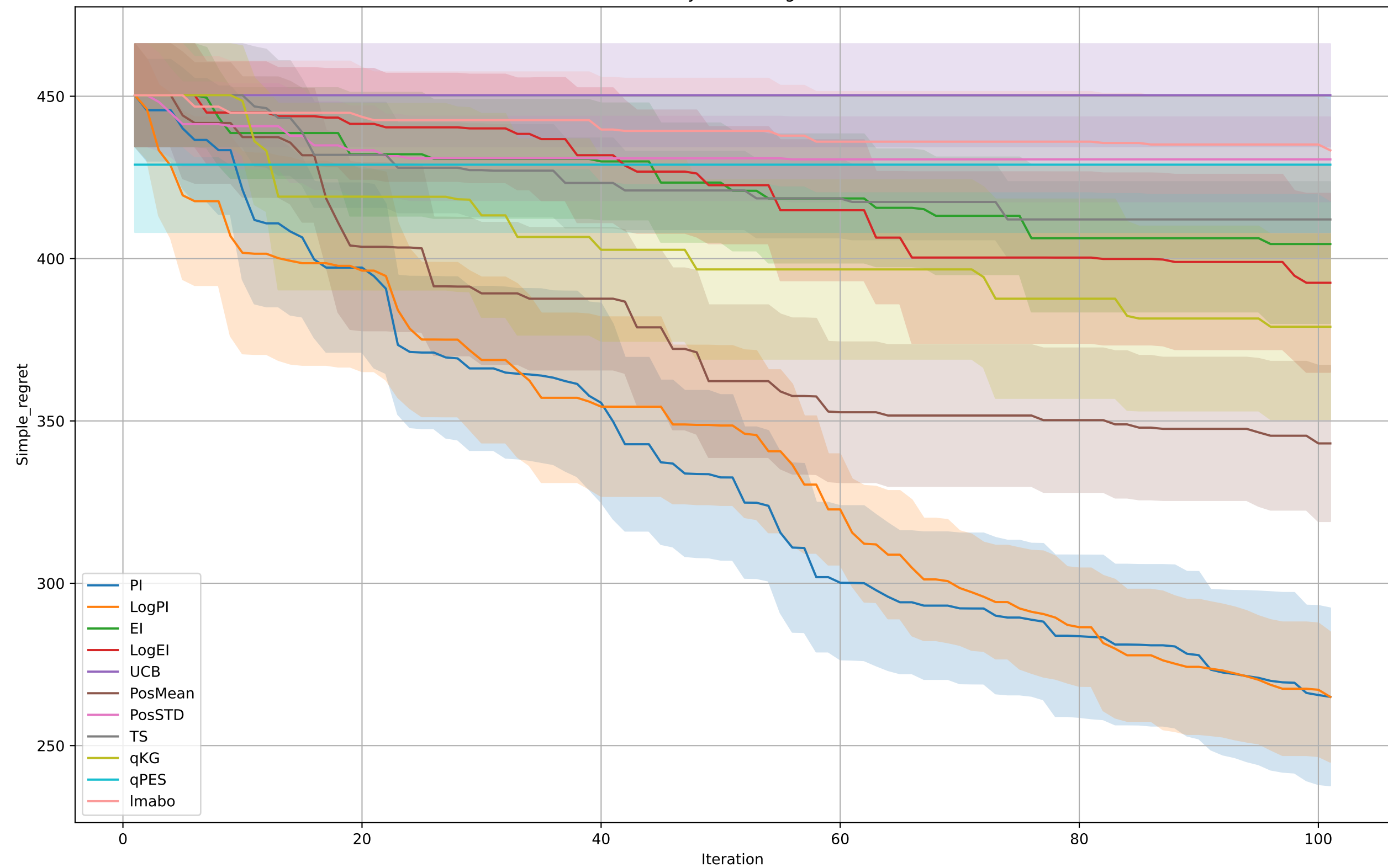
StyblinskiTang
