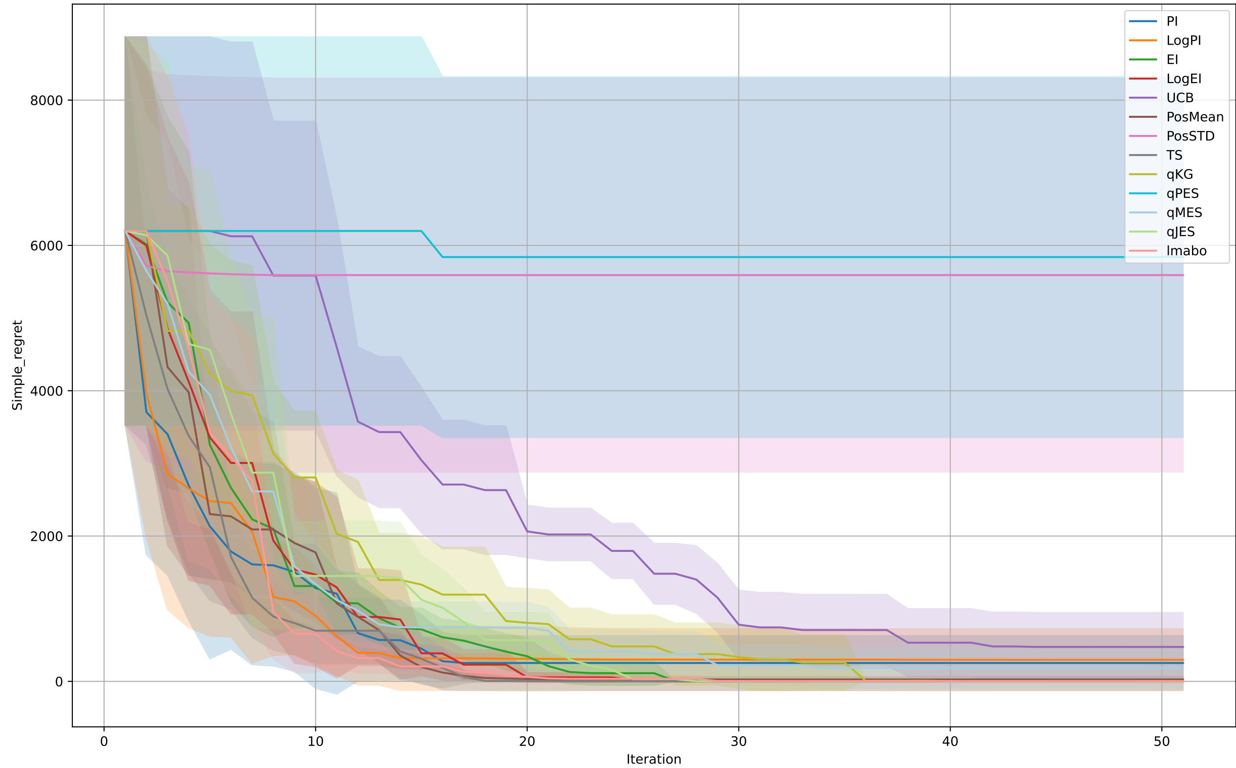
Schwefel
