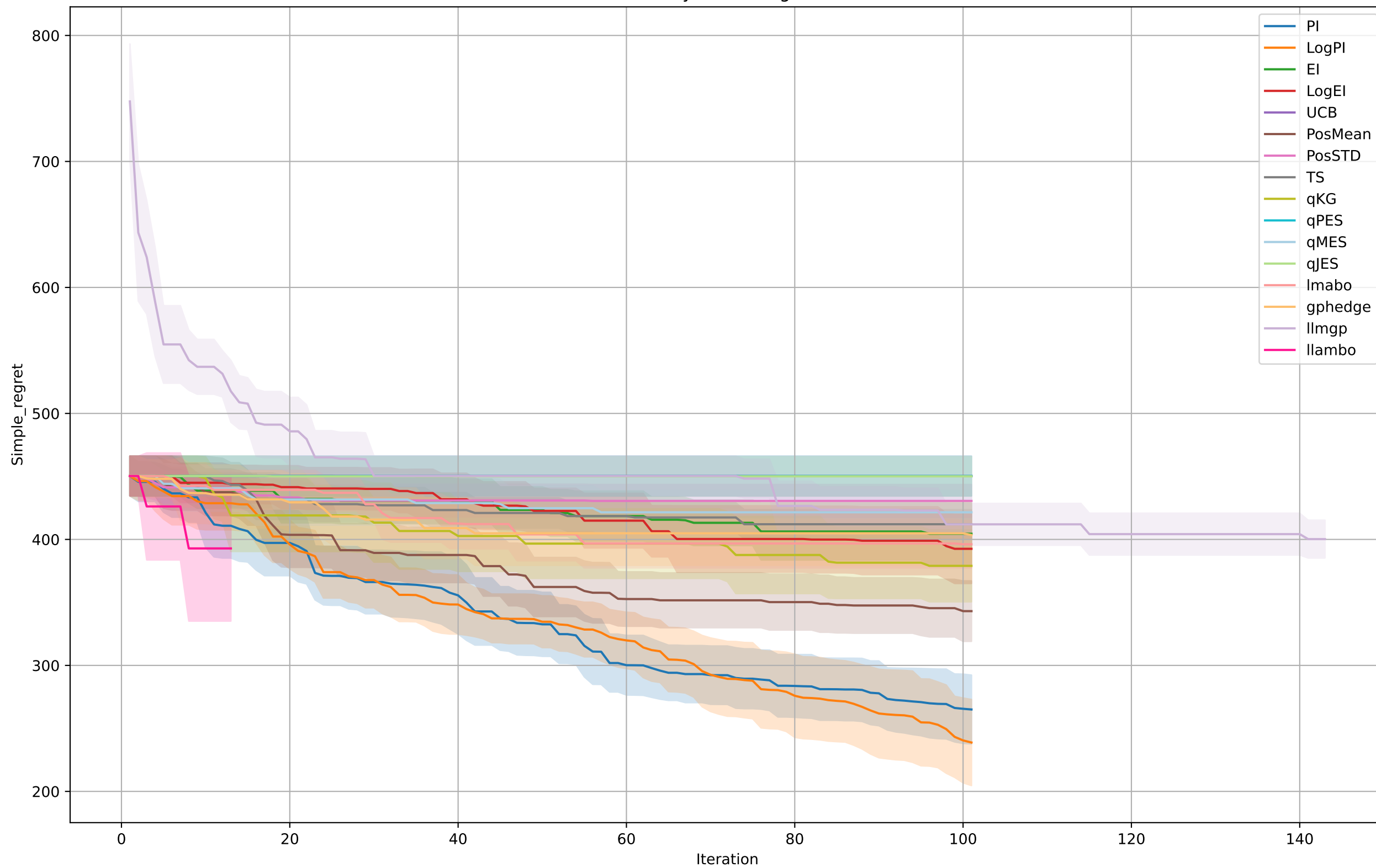
StyblinskiTang
