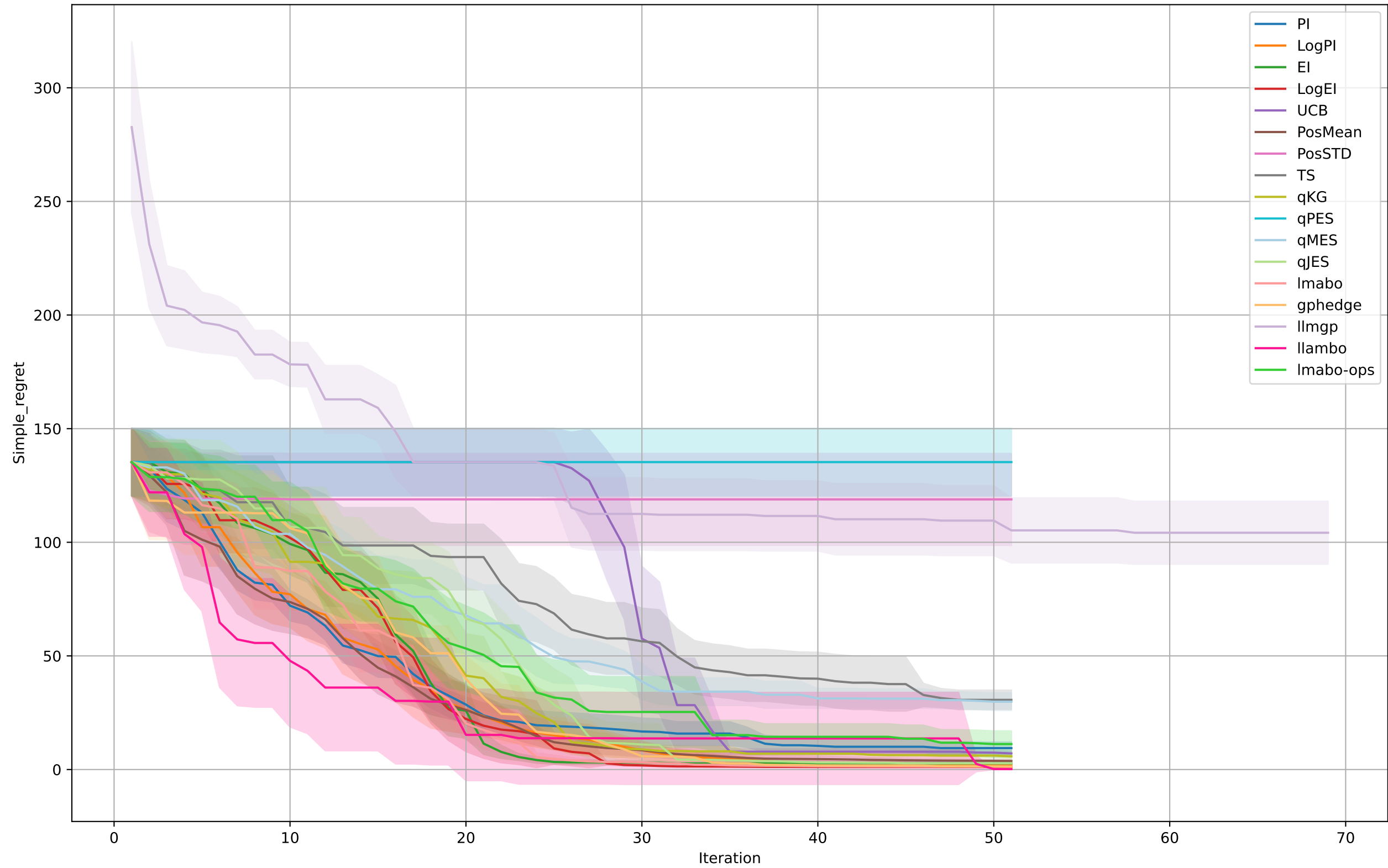
Griewank
