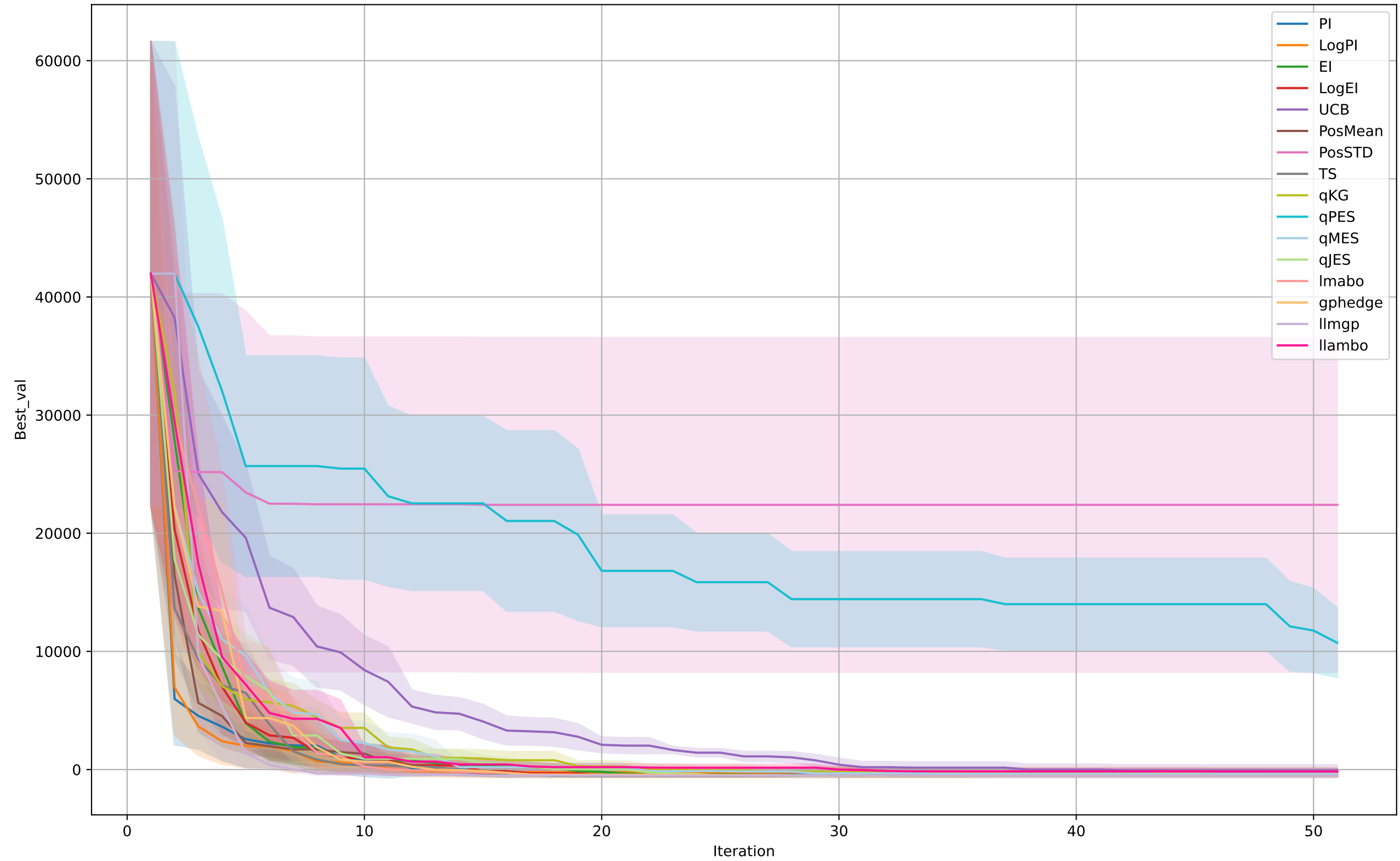
Schwefel
