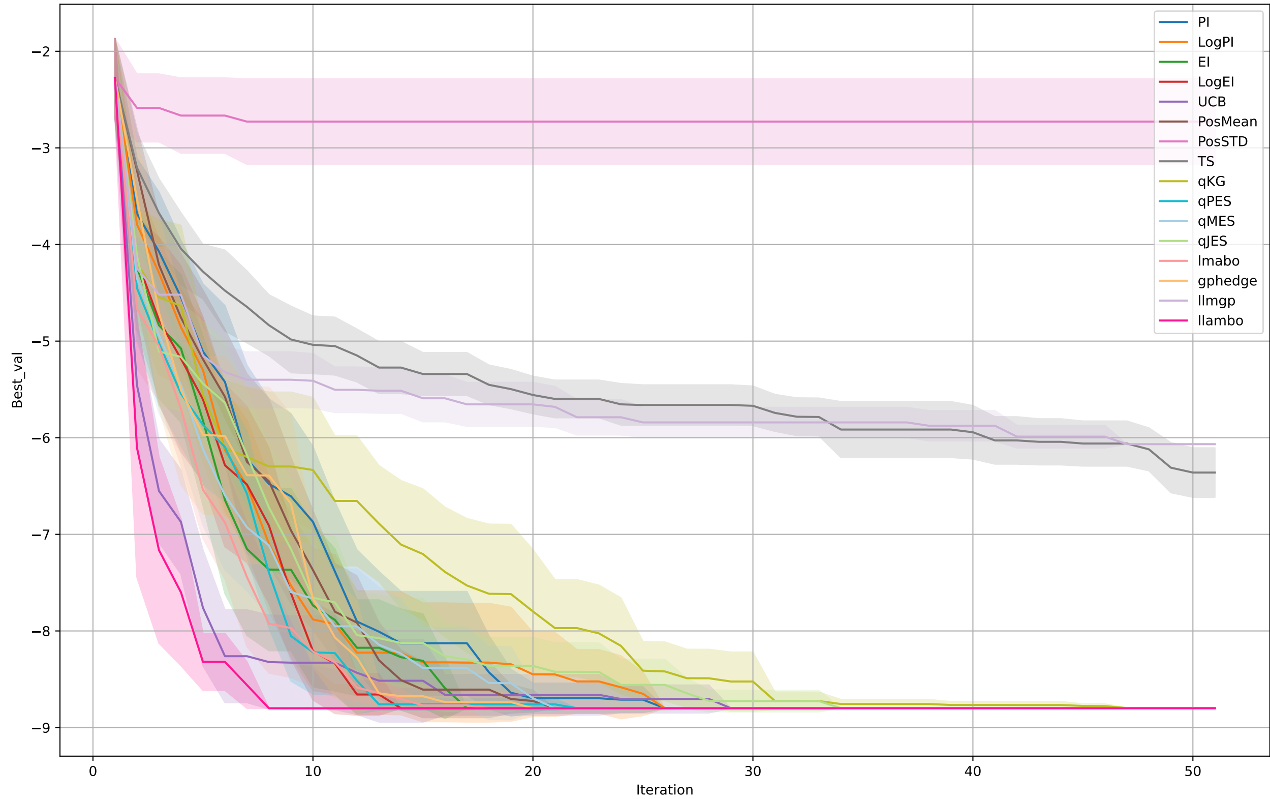
Cosine8
