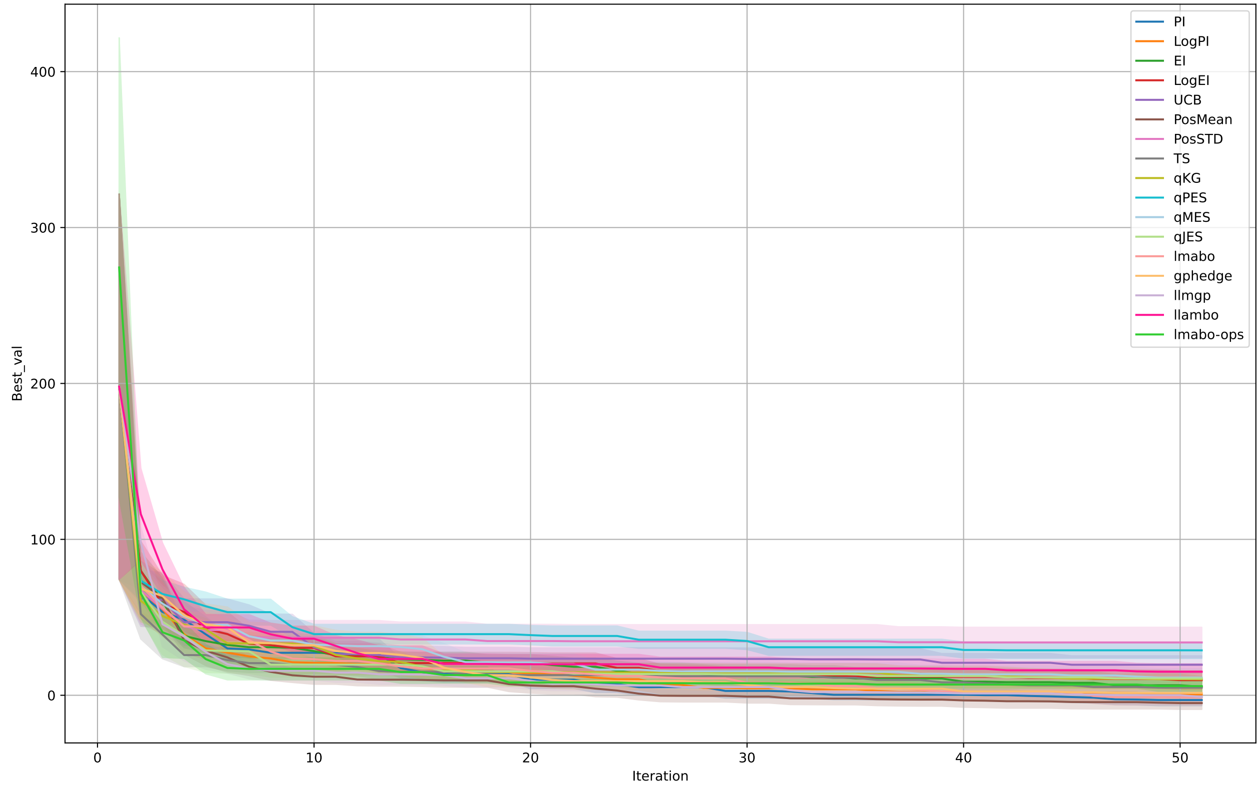
SchaffersIIICond
